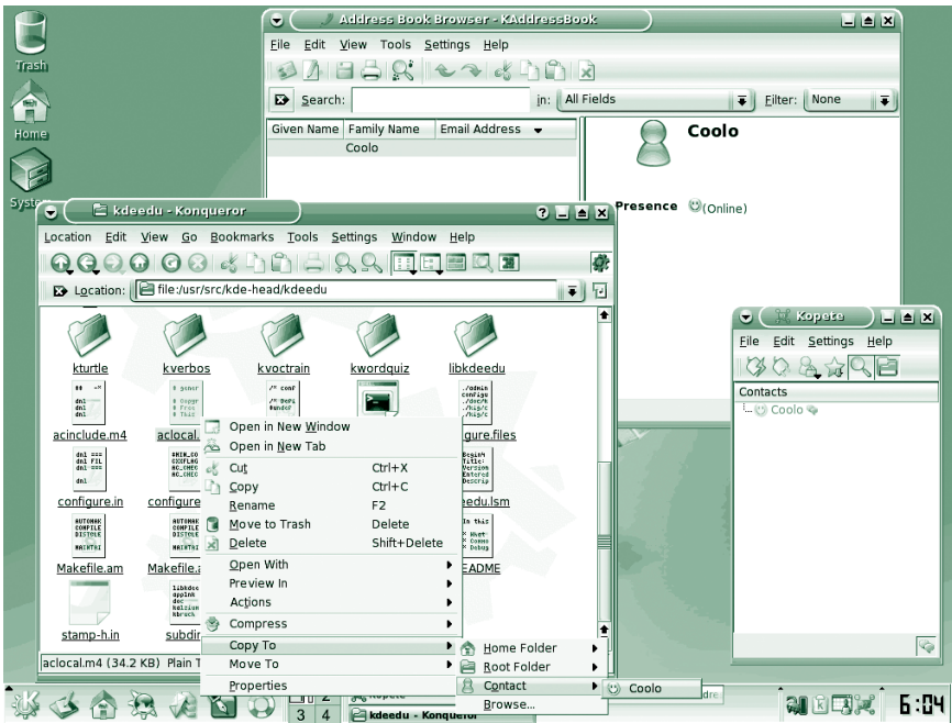
Abbildung 10.2: KDE-Oberfläche
