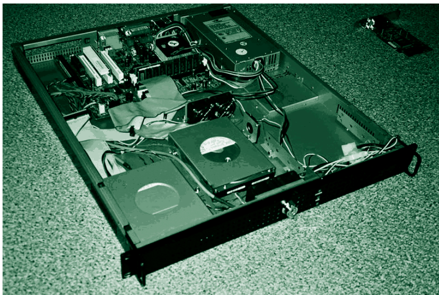
Abbildung 9.4: Typischer Root-Server in moderner Flachbauweise für Einbau in 19«-Racks
