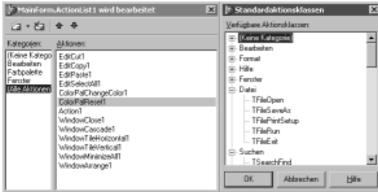
Abbildung 4.9: Zusammenstellen eigener Aktionslisten (links) aus den mit der VCL mitgelieferten Standardaktionen (rechts). Die beiden ColorPal...-Aktionen sind in der Komponentenbibliothek dieses Buchs definiert (Kategorie »Farbpalette«).
