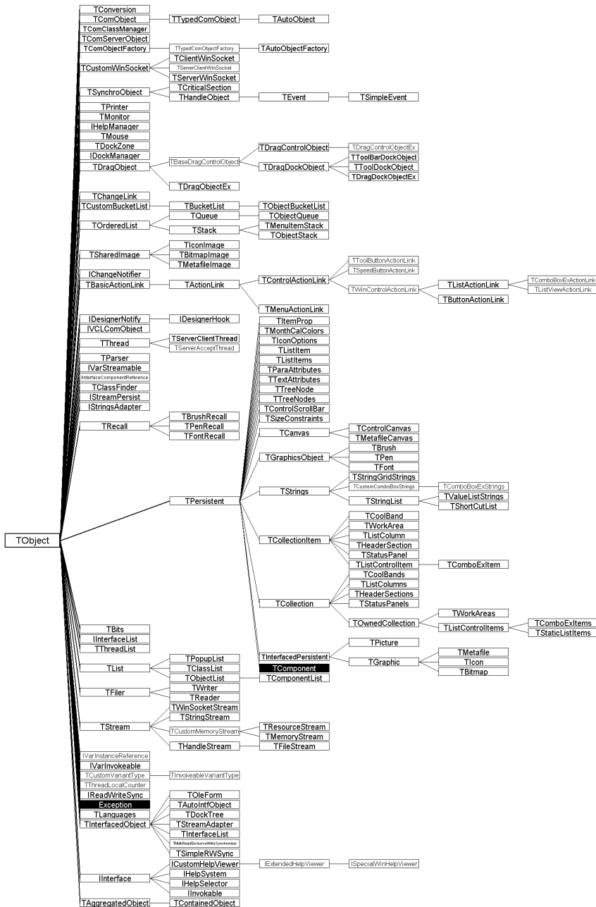
Abbildung B.1: Die »Wurzelregion« der VCL-Klassenhierarchie, aus Platzgründen hier beschränkt auf eine Auswahl von Klassen der Personal-Ausgabe (für eine umfassende Übersicht bedarf es eines großen Posters, wie es von Borland mitgeliefert wird).
