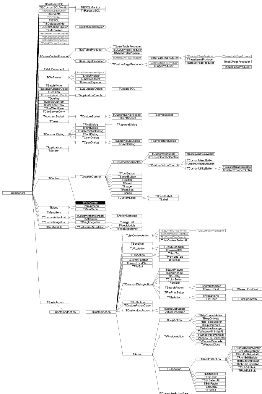
Abbildung B.2: TComponent bildet die Grundlage für alle Komponenten, sowohl visuelle als auch nicht-visuelle (hier auch mit Klassen aus Professional- und Enterprise-Version).
