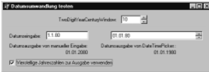
Abbildung 2.2: Ein Testprogramm für die Datumsumwandlung zeigt, dass die TDateTimePicker -Komponente bei zweistelliger Jahreseingabe das TwoDigitYearCenturyWindow nicht beachtet.
