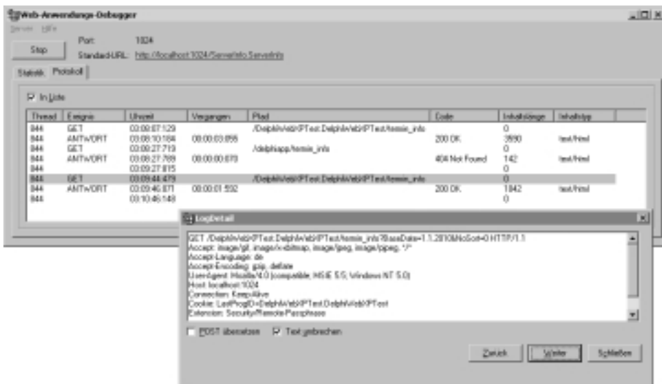
Abbildung 8.28: Der Web-Anwendungs-Debugger beim Protokollieren des bei der Nutzung des Beispielperogramms entstehenden HTTP-Verkehrs
