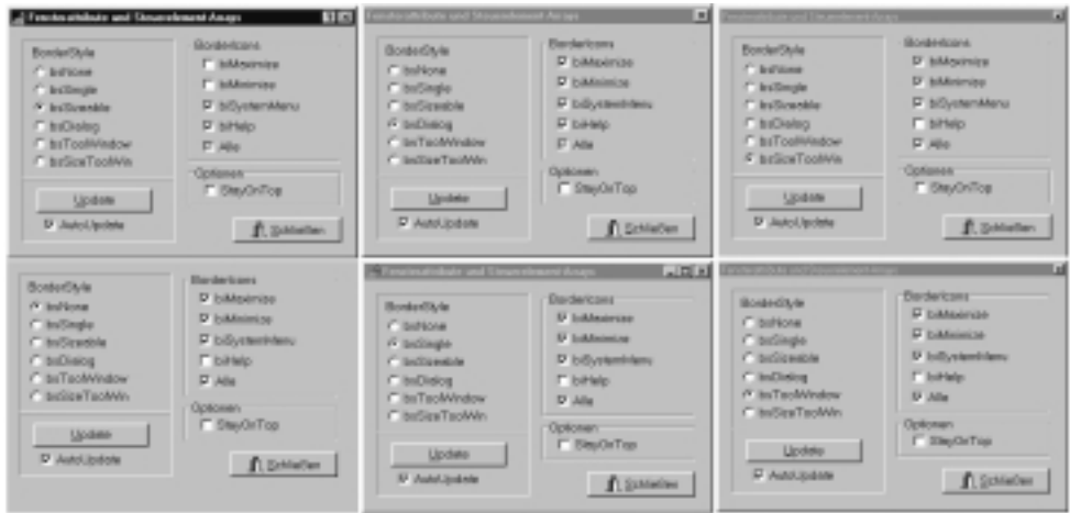
Abbildung 3.4: Verschiedene Formularstile, demonstriert von StyleBtn
