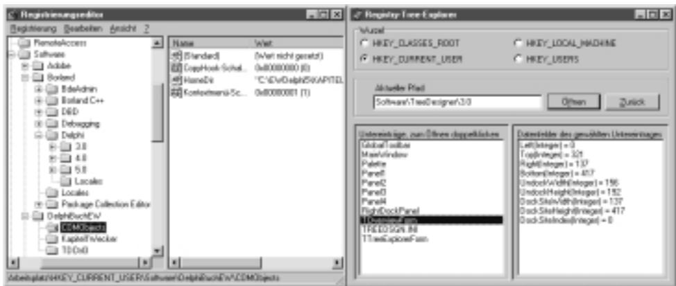
Abbildung 4.1: Der Registrierungseditor von Windows 95 und das Beispielsprogramm RegBrows zum Browsen durch die Registry
