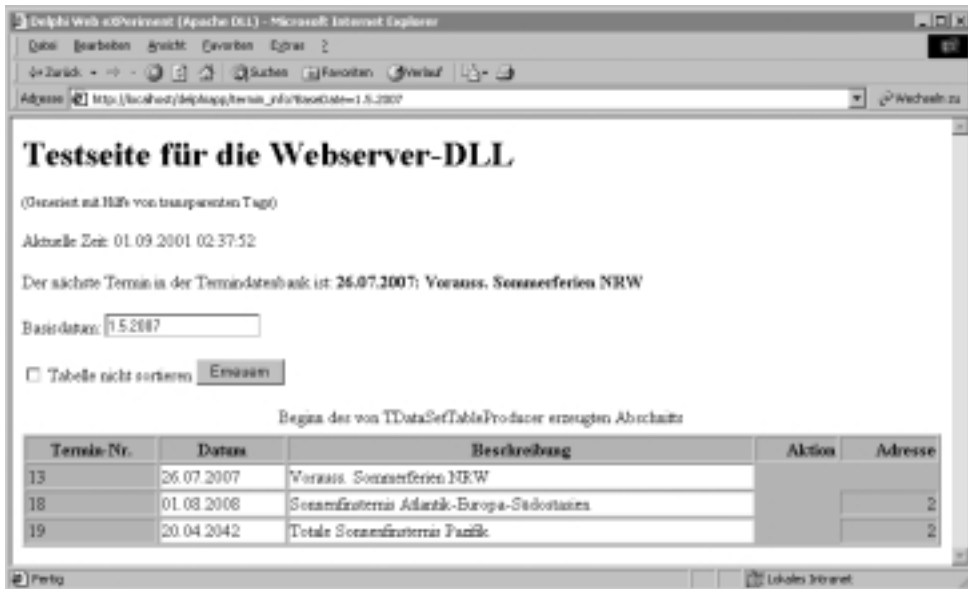
Abbildung 8.27: Die erweiterte Datenbankseite enthält ein HTML-Formular zur Einstellung der Parameter der HTTP-Anfrage.
