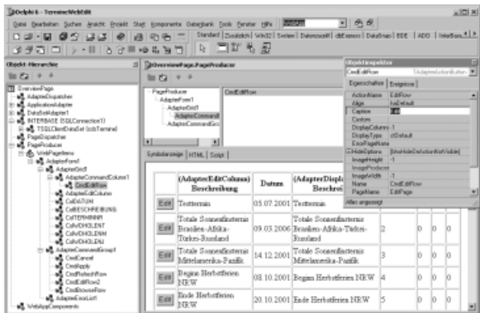
Abbildung 8.32: Die Objekt-Hierarchie der Tabellenseite (OverviewPage) und der dafür zuständige Seiteneditor
