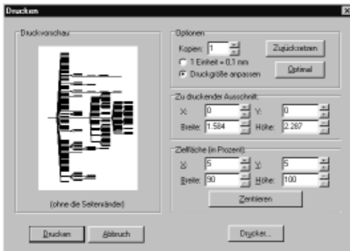
Abbildung 5.9: Nach Drücken des Schalters »Optimal«, Verkleinern der Zielfläche auf 90% und Verschieben der Zielfläche um jeweils 5% in X- und Y-Richtung wird diese Grafik zentriert gedruckt und füllt die Seite fast ganz aus.
