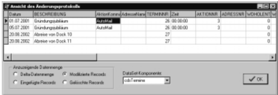
Abbildung 7.24: Ansicht der geänderten Datensätze über die ClientDataSet -Option »StatusFilter = usModified«. Jeder geänderte Datensatz wird zwei Mal angezeigt: einmal für den Zustand vor der Änderung, einmal für den Zustand danach.
