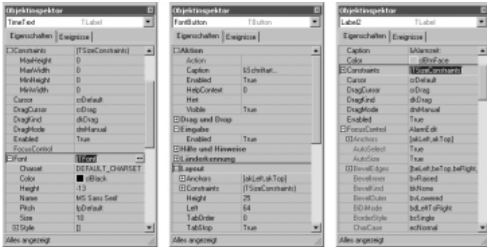
Abbildung 1.4: Geschachtelte Properties und nach Kategorien sortierte Properties, rechts in Delphi 6 neu eingeführte Darstellung von Properties einer verknüpften Komponente (hier TLabel.FocusControl)
