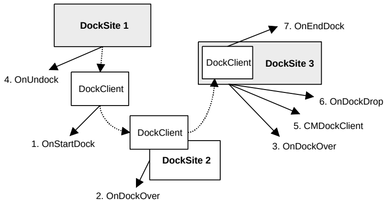
Abbildung 5.12: Die Ereignisse beim Drag&Dock eines andockbaren Fensters (DockClient) von einer ersten Andockstelle (DockSite1) über eine zweite hinweg bis zu einer dritten, über der die Maustaste losgelassen wird.
