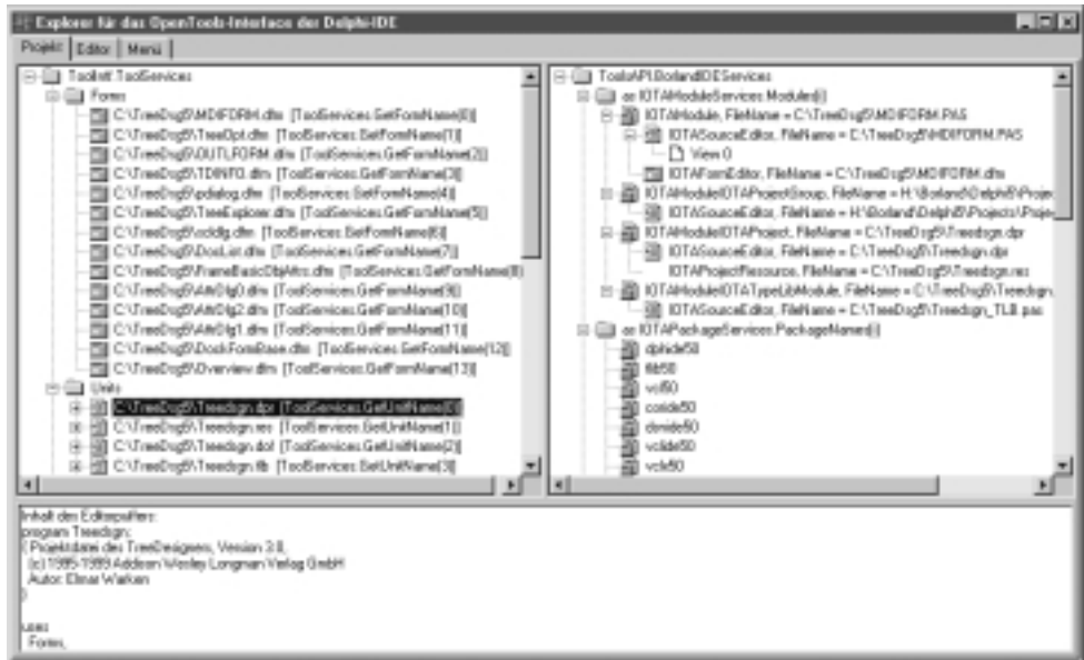
Abbildung A.2: Diese beiden TreeViews des ToolsAPI-Explorers zeigen gewissermaßen die »Besitzhierarchie« der ToolsAPI-Schnittstellen: links die Informationen der in allen Delphi-Versionen bekannten ToolServices, rechts die der neueren BorlandIDEServices.
