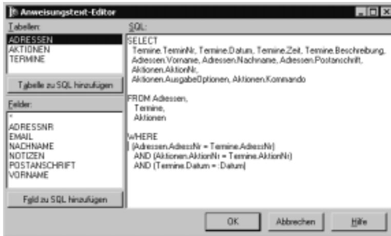
Abbildung 7.20: Eingabe von SQL-Anweisungen für dbExpress-Komponenten
