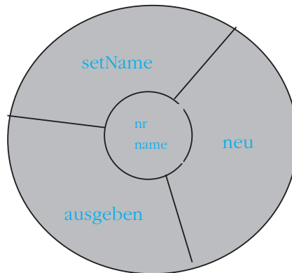
Abb. 11.2: Klasse Partner01 als Doughnut-Diagramm
