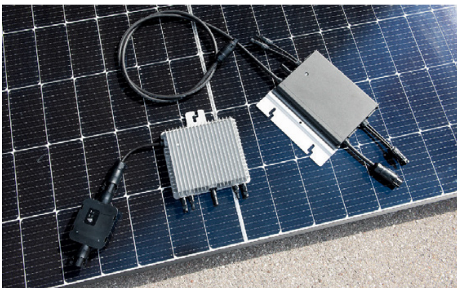
Wechselrichter. Drei Geräte nutzen den problematischen von Hoymiles (rechts). Der von Deye (links) stört Funk kaum.
