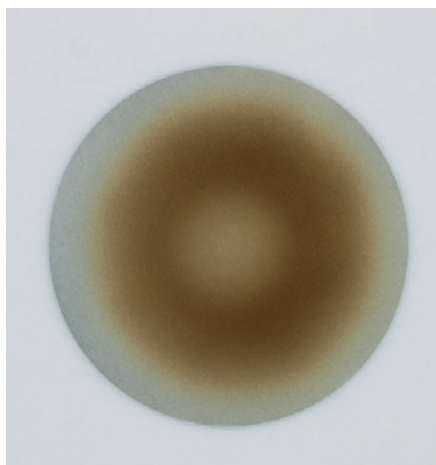
Temperaturverteilung. Das gebräunte Mehl auf der Metallplatte zeigt die Kontur der Induktionsspule. Im Beispiel rechts laufen zwei ovale Spulen unter der Kochstelle entlang.
