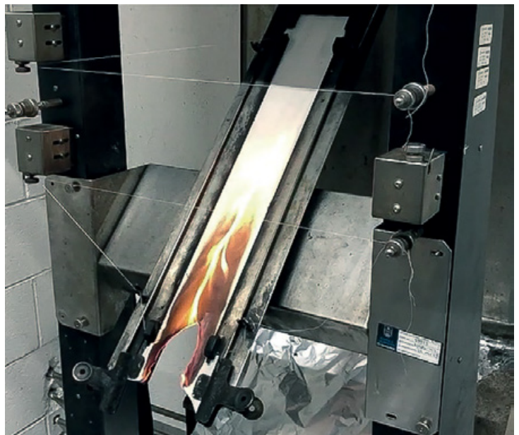
In Flammen. Auf dem Matratzenbezug von Nuna breitete sich das Feuer zu schnell aus.
