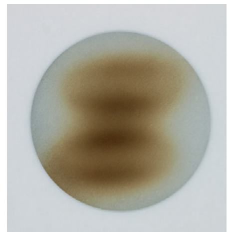
Temperaturverteilung. Das gebräunte Mehl auf der Metallplatte zeigt die Kontur der Induktionsspule. Im Beispiel rechts laufen zwei ovale Spulen unter der Kochstelle entlang.
