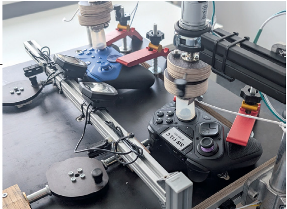
Eigenkreation. Unsere selbst gebaute Maschine malträtierte die Controller im Dauertest millionenfach.
