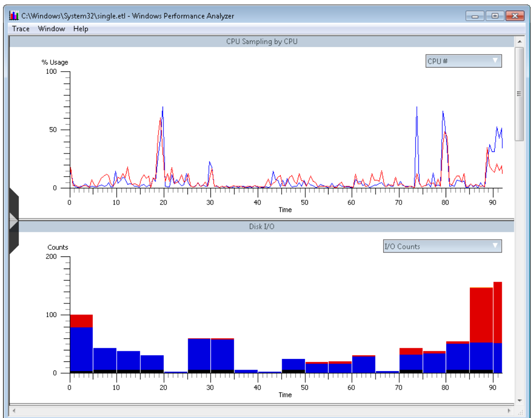
Abbildung 13.52 Aufgezeichnete Ablaufverfolungsdaten im Performance Analyzer
