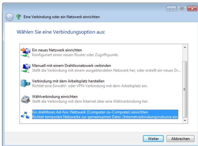
Abbildung 6.45 Auswählen der Option Ein drahtloses Ad-hoc-Netzwerk (Computer-zu-Computer) einrichten
