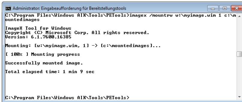
Abbildung 3.16 Bereitstellen eines WIM-Abbilds im Dateisystem mit ImageX
