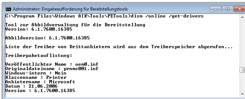
Abbildung 3.7 Auflisten der Treiber im Onlinesystemabbild
