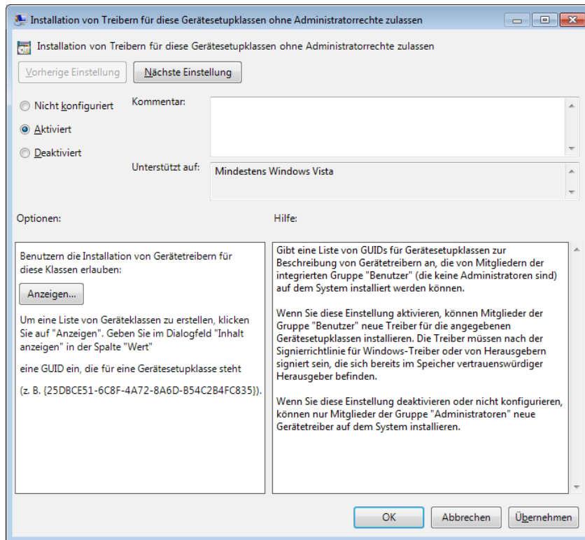
Abbildung 4.26 Aktivieren der Richtlinie Installation von Treibern für diese Gerätesetupklassen ohne Administratorrechte zulassen
