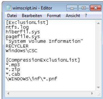
Abbildung 2.7 Eine Wimscript.ini -Datei
