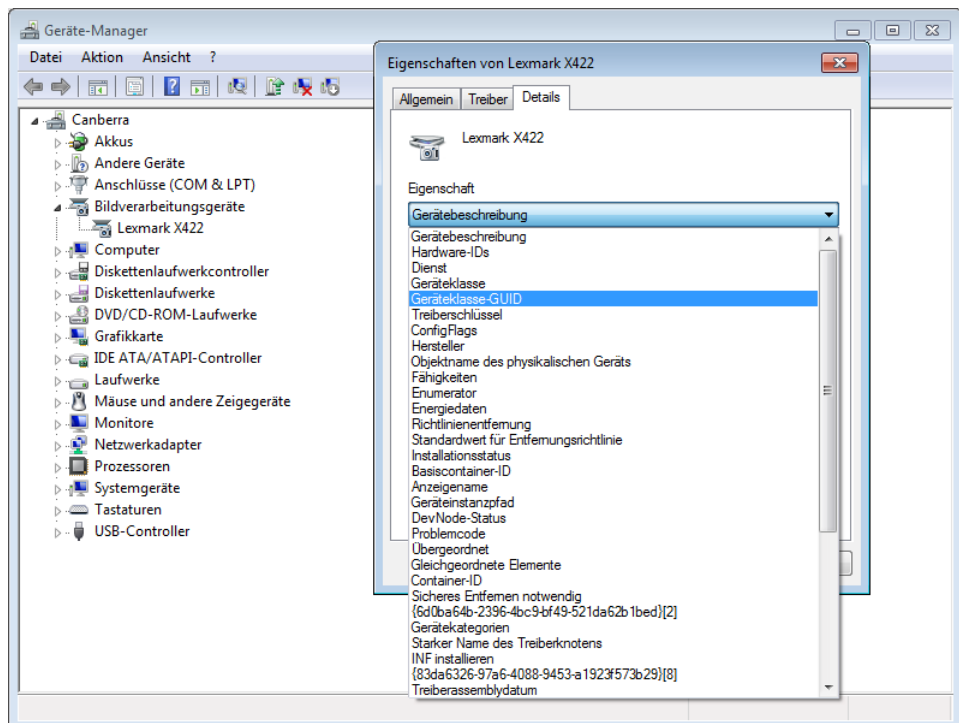
Abbildung 4.23 Ermitteln einer Geräteklassen-GUID
