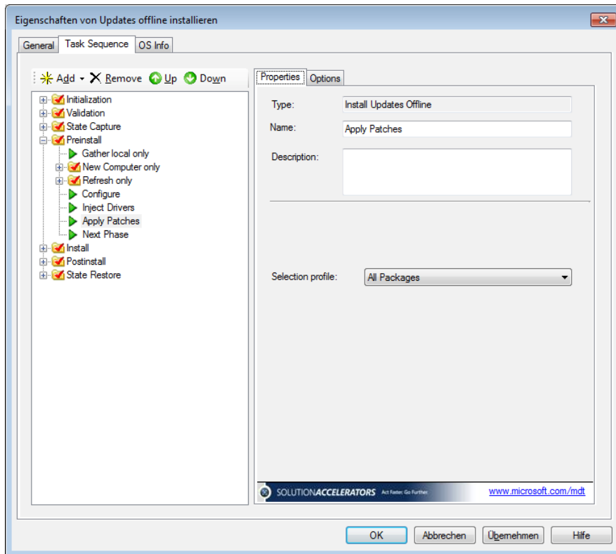
Abbildung 3.25 Die Vorlage Standard Client Task Sequence
