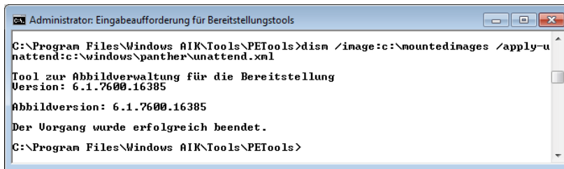
Abbildung 3.14 Anwenden einer Antwortdatei auf ein offline bereitgestelltes Abbild
