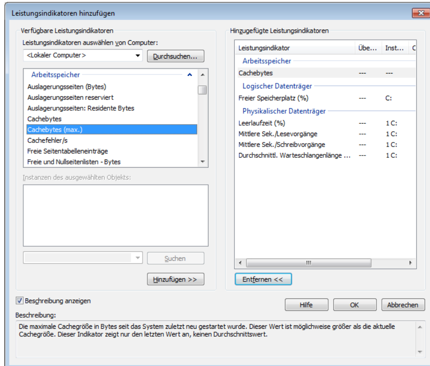
Abbildung 13.25 Die benötigten Leistungsindikatoren und Instanzen wurden ausgewählt
