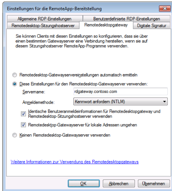
Abbildung 10.19 Remotedesktopgatewayeinstellungen für RemoteApp
