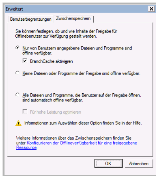
Abbildung 8.42 Aktivieren von BranchCache für eine Freigabe
