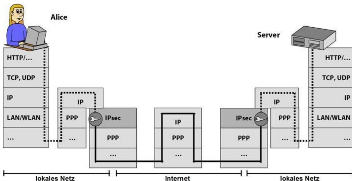
Abb. 41–2 IPsec kann auch als Tunnel-Protokoll für ein VPN verwendet werden. Dabei werden IPPakete innerhalb von IP-Paketen übertragen.
