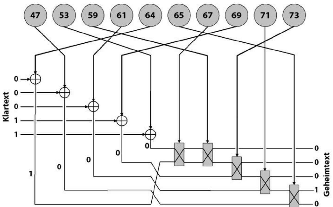
Abb. 5–14 Der Geheimschreiber arbeitete mit zehn gezahnten Rädern. Fünf davon beeinflussten den Klartext direkt, die anderen fünf sorgten für eine zusätzliche Durchmischung.
