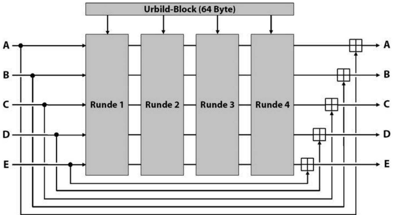
Abb. 16–2 Die Kompressionsfunktion von SHA-1 arbeitet in vier Runden.
