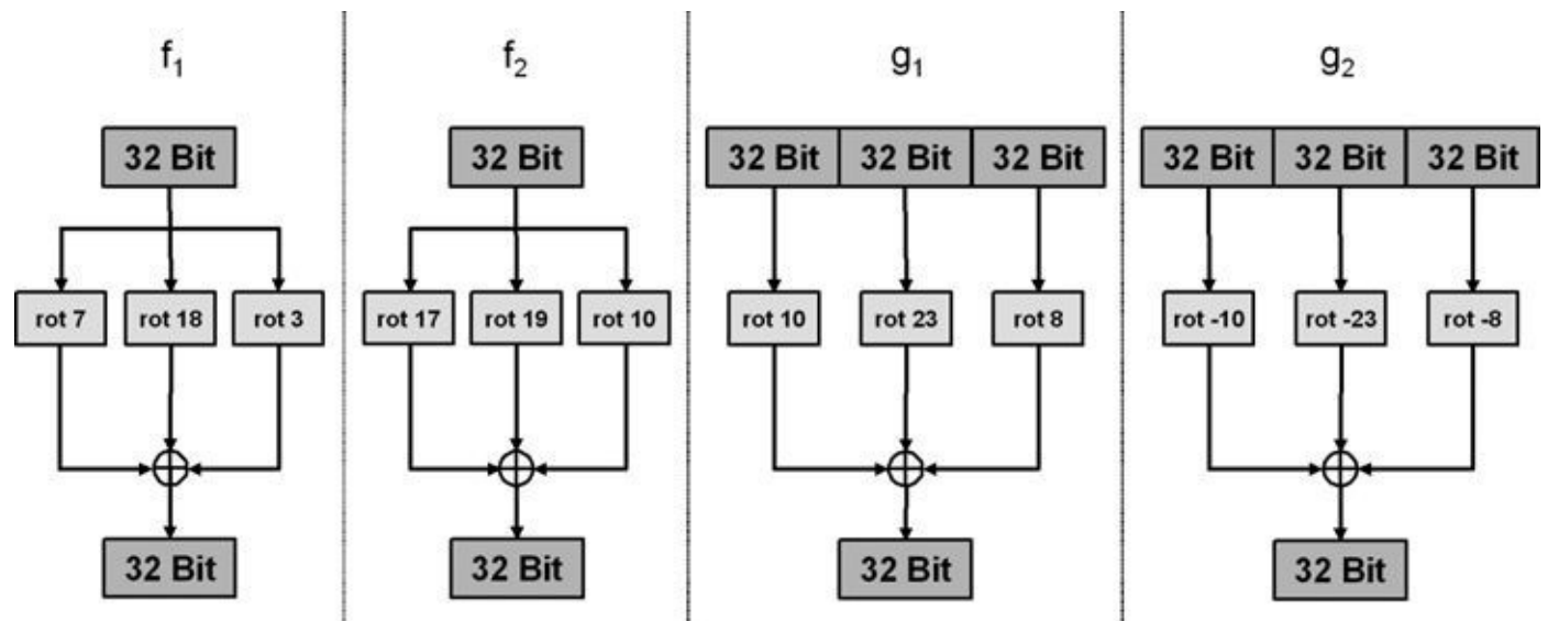
Abb. 21–5 Für die Funktionsweise von HC-128 spielen die Funktionen f_1, f_2, g_1 , und g_2 eine Rolle.
