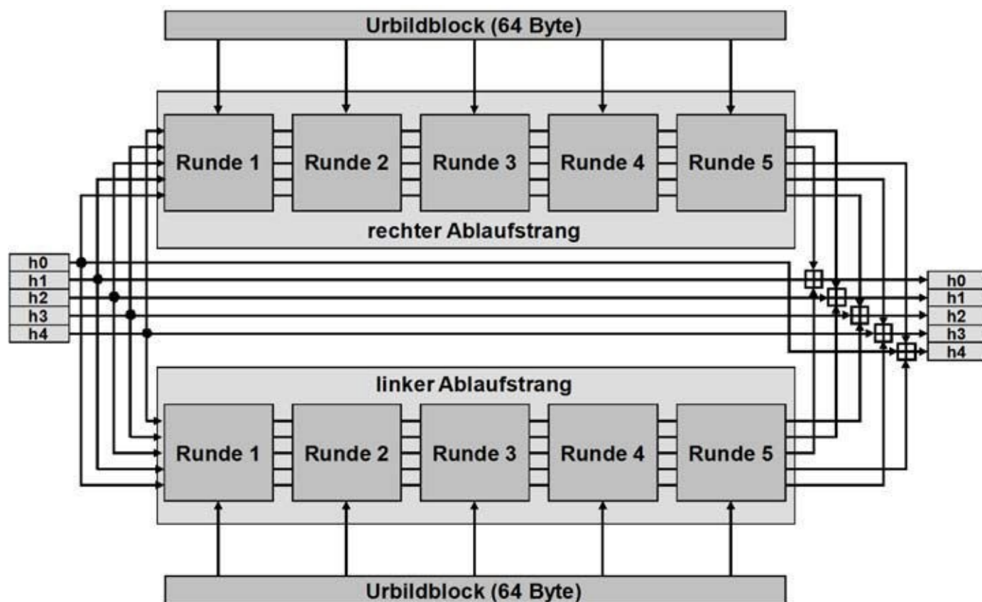
Abb. 16–5 Die Kompressionsfunktion von RIPEMD-160 arbeitet in zwei parallelen Ablaufsträngen.
