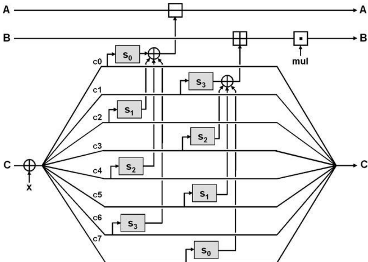
Abb. 17-4 Eine Teilrunde (round) von Tiger. s_0 , s_1 , s_2 und s_3 sind S-Boxen.
