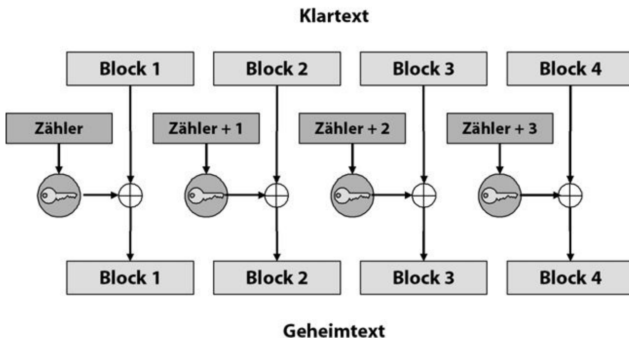
Abb. 24-6 Der Counter-Modus ist der Shooting-Star unter den Betriebsarten.
