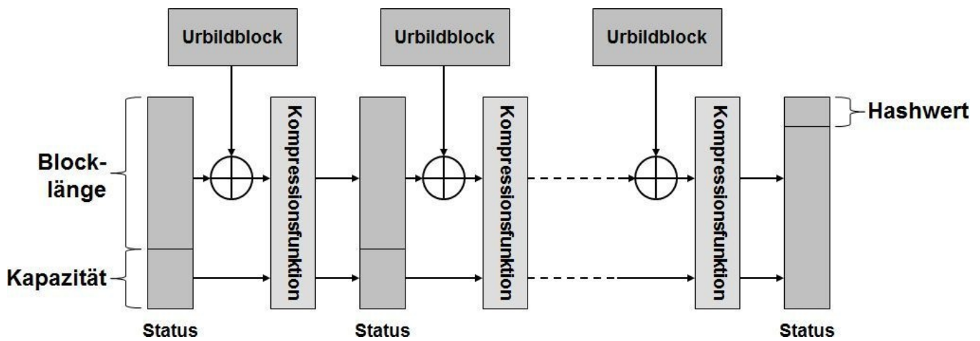
Abb. 17–7 Das Funktionsprinzip von Keccak wird auch als Schwamm bezeichnet. Die Länge des Hashwerts entspricht der Hälfte der Kapazität.
