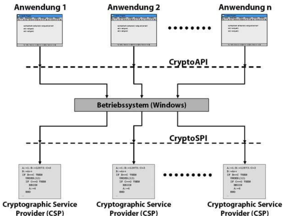
Abb. 31-2 Die MS-CAPI ist in das Windows-Betriebssystem integriert.
