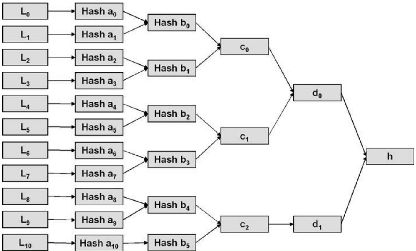
Abb. 18–1 Durch den Einsatz von Hashbäumen benötigt man nicht den gesamten signierten Text, um eine digitale Signatur zu verifizieren.
