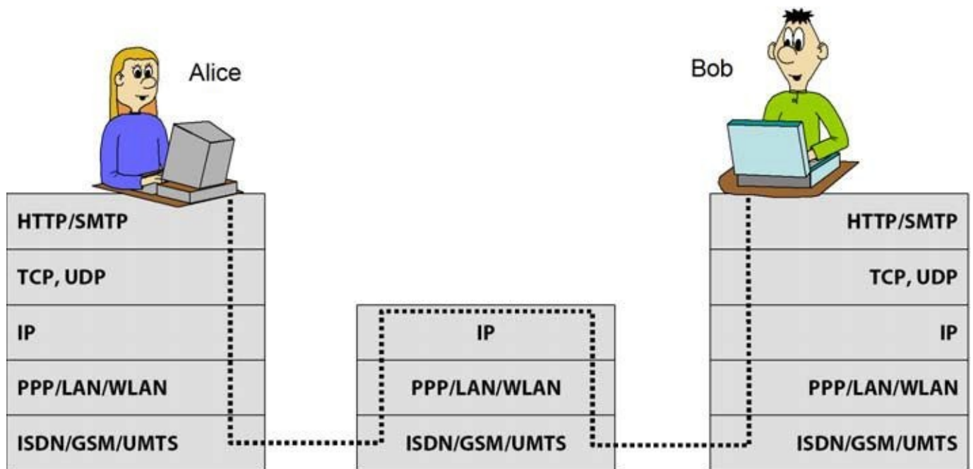
Abb. 38–2 Eine Kommunikation im Internet läuft über einen oder mehrere Router. In einem Router ist IP die höchste Schicht.
