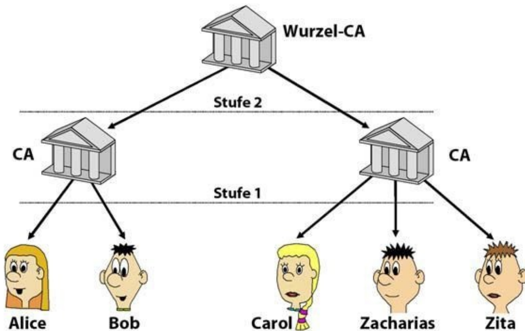
Abb. 33–7 Beispiel für eine zweistufige CA-Hierarchie
