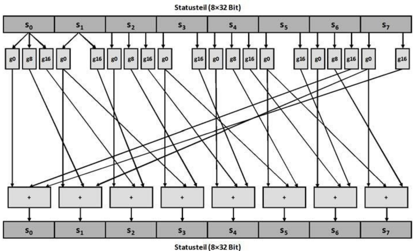
Abb. 21–8 Die Fortschaltung des Statusteils von Rabbit erfolgt mit nichtlinearen Funktionen.
