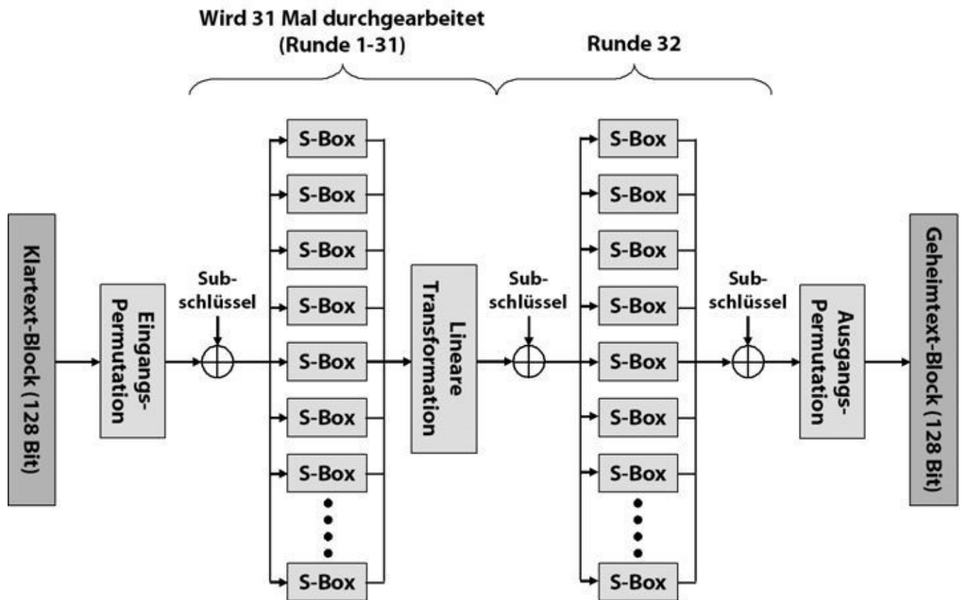
Abb. 11–1 Serpent arbeitet in 32 Runden, wobei die letzte einen leicht geänderten Ablauf hat.
