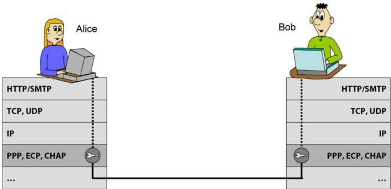
Abb. 40–1 ECP (Verschlüsselung) und CHAP (Authentifizierung) sichern Schicht 2 des OSI-Modells kryptografisch ab.
