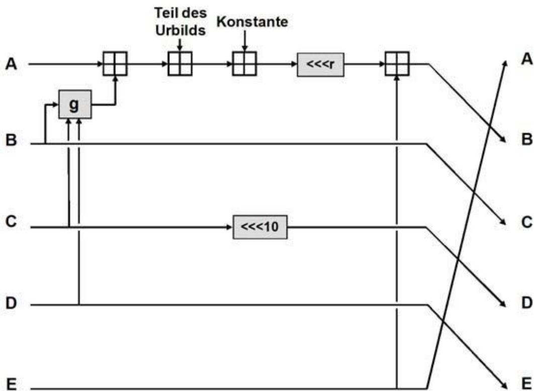
Abb. 16-6 Jede RIPEMD-160-Runde sieht 16 dieser Operationen vor. Die Konstante und die Funktion g sind von der jeweiligen Runde abhängig.
