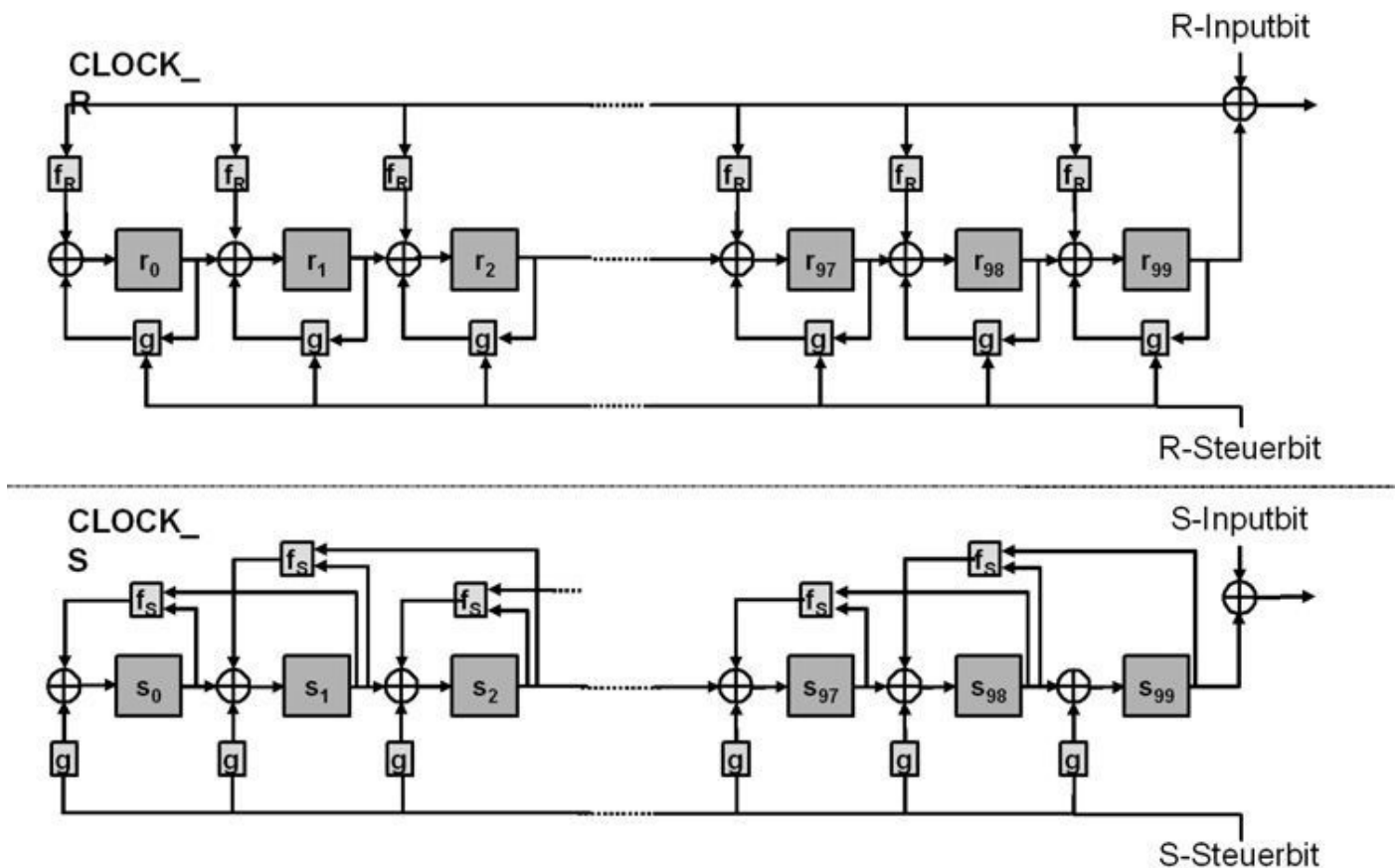
Abb. 21–14 Die für Hardwareumsetzungen optimierte Stromchiffre MICKEY arbeitet mit den beiden Funktionen CLOCK_R und CLOCK_S .
