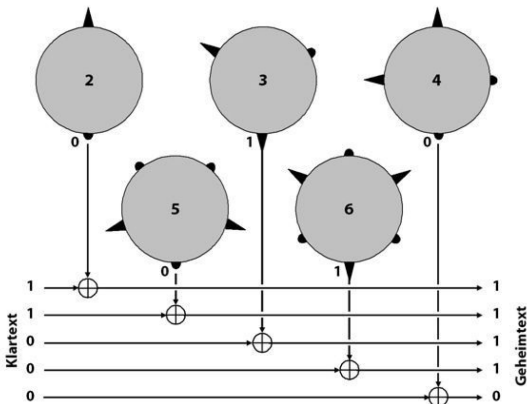
Abb. 5-13 Vereinfachte Variante eines Geheimschreibers: Fünf gezahnte Räder bilden ein Muster von Nullen und Einsen, die mit dem Klartext exklusiv-oder-verknüpft werden.
