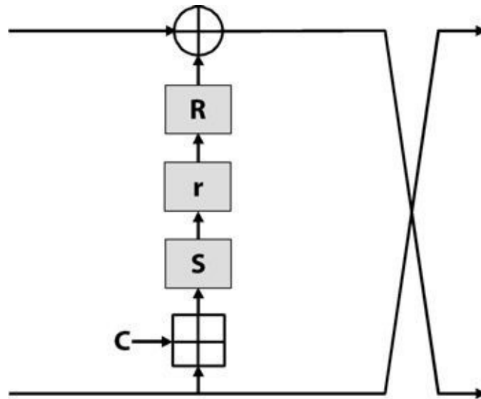
Abb. 12–6 Die SEA-Schlüsselaufbereitung generiert für jede Runde einen Subschlüssel.
