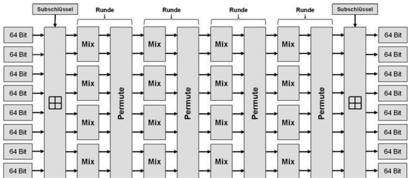
Abb. 12–8 Threefish arbeitet in 72 oder 80 Runden. Vier davon sind hier zu sehen.
