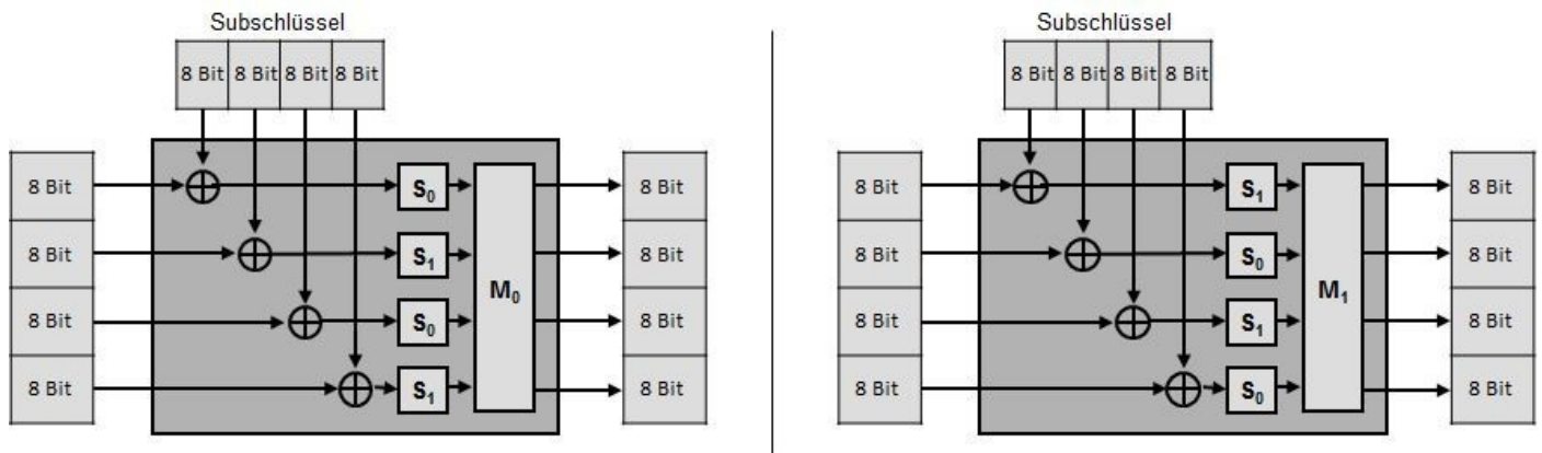
Abb. 12-4 Die Funktionen F_0 (links) und F_1 (rechts) sind die zentralen Bausteine von CLEFIA.
