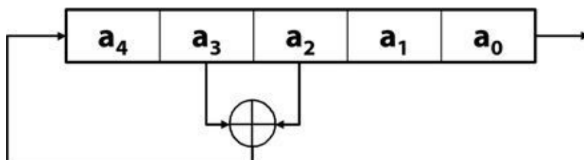
Abb. 19–3 Beispiel für ein linear rückgekoppeltes Schieberegister (LFSR). a_2 und a_3 sind die Tap-Variablen.
