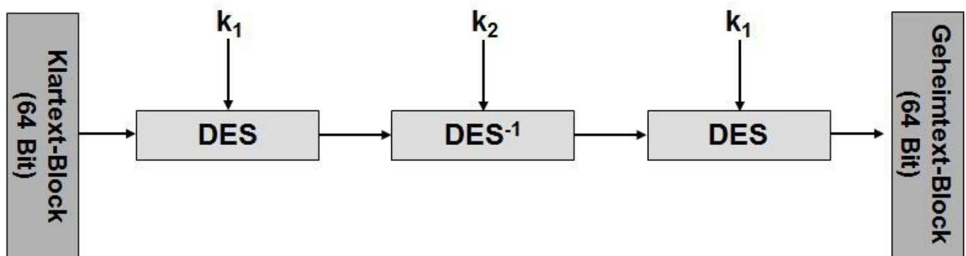
Abb. 6–4 Beim Triple-DES wird der DES dreimal hintereinander angewendet (meist mit nur zwei Schlüsseln). Die mittlere Anwendung ist eine Entschlüsselung.
