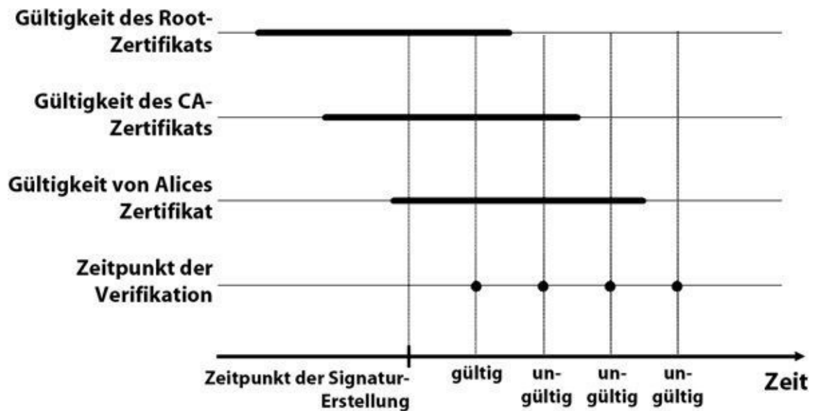
Abb. 36–1 Im PEM-Schalenmodell ist eine Signatur gültig, wenn zum Verifikationszeitpunkt sowohl Alices Zertifikat als auch das CA-Zertifikat als auch das Wurzel-CA-Zertifikat gültig sind.
