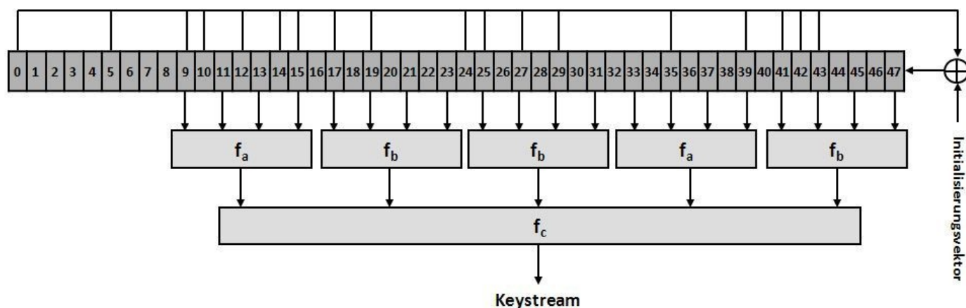
Abb. 21–4 Crypto1 ist eine einfache und nicht besonders sichere Stromchiffre.
