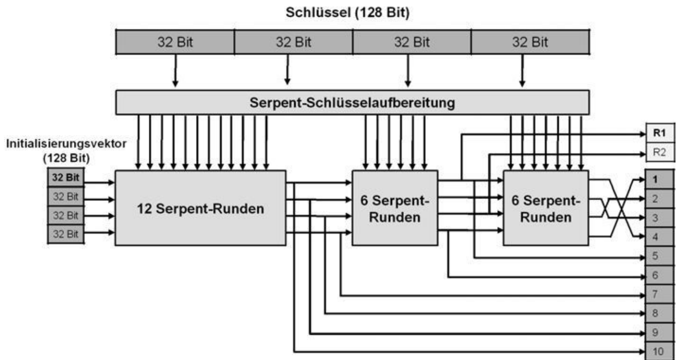
Abb. 21–11 So werden die 12 Statusvariablen von Sosemanuk initialisiert.
