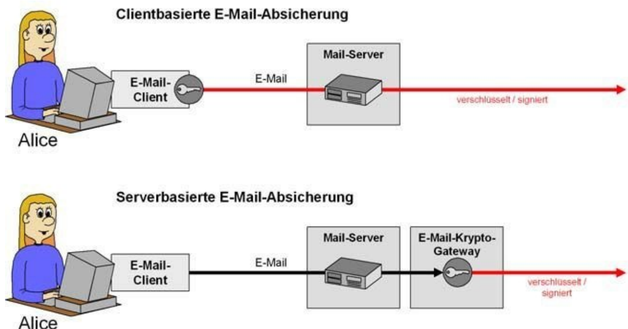
Abb. 43–1 Bei der clientbasierten E-Mail-Absicherung übernimmt Alice selbst das Verschlüsseln und Signieren. Bei der serverbasierten Variante überlässt sie diese Aufgaben einem E-Mail-Krypto-Gateway.
