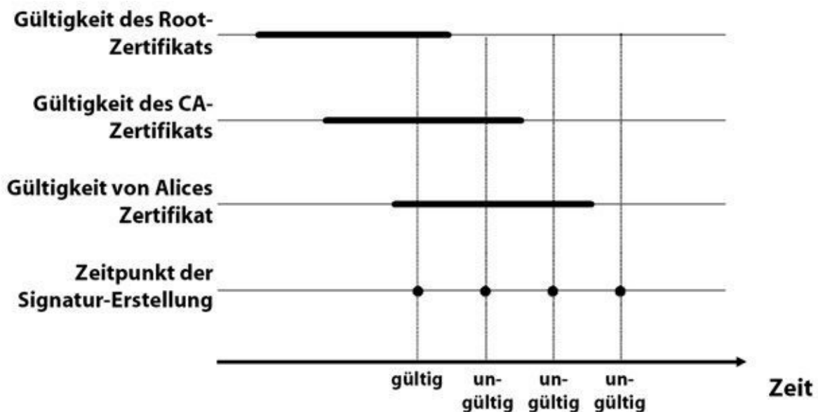
Abb. 36–2 Im modifizierten Schalenmodell ist eine Signatur dann gültig, wenn zum Signierzeitpunkt alle beteiligten Zertifikate gültig sind.
