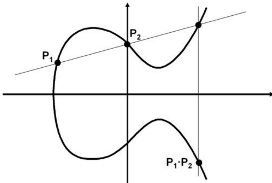
Abb. 15–2 Zwei Punkte einer elliptischen Kurve werden multipliziert, indem eine Gerade durch sie gezogen wird. Das Ergebnis ist die Spiegelung des dritten Schnittpunkts an der x -Achse.
