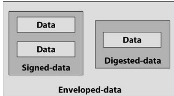
Abb. 23–1 PKCS#7 beschreibt ein rekursives Format für verschlüsselte, signierte und gehashte Daten. In diesem Bild sind eine signierte und eine gehashte Einheit in einer verschlüsselten enthalten.
