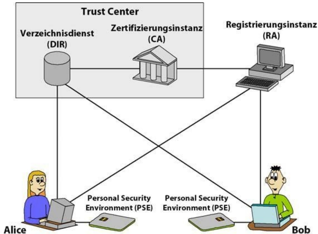
Abb. 33–10 Aufbau einer PKI: Die zentralen Komponenten werden im Trust Center zusammengefasst. Die PCs von Alice und Bob sind Beispiele für Endeinheiten. Die Speicherung der privaten Schlüssel erfolgt im PSE, das etwa als Smartcard realisiert sein kann.
