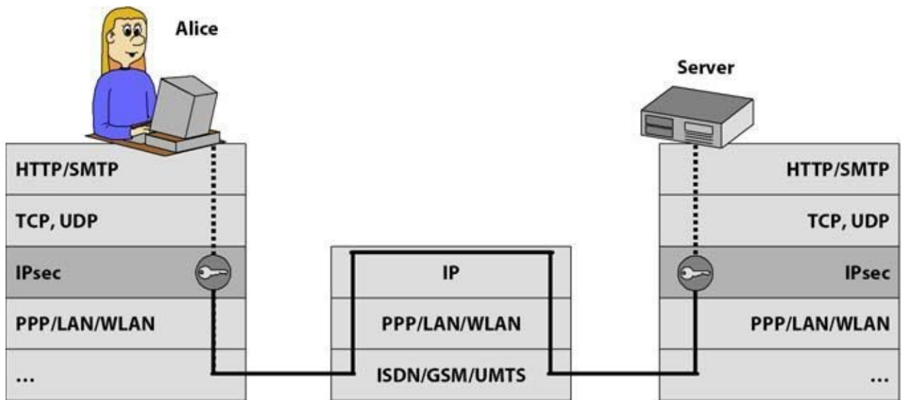
Abb. 41–1 IPsec ermöglicht den Einsatz von Kryptografie in Schicht 3 des OSI-Modells. Mit IPsec kann auch nur eine Teilstrecke des Internets kryptografisch abgesichert werden.
