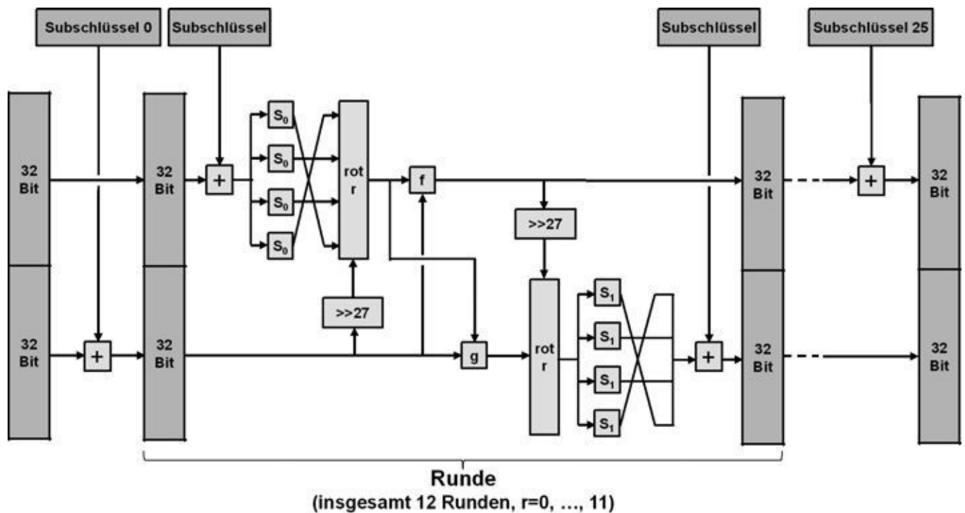
Abb. 12-2 Chiasmus ist eine SP-Chiffre. Das Verfahren wird von deutschen Behörden und deren Kommunikationspartnern eingesetzt.
