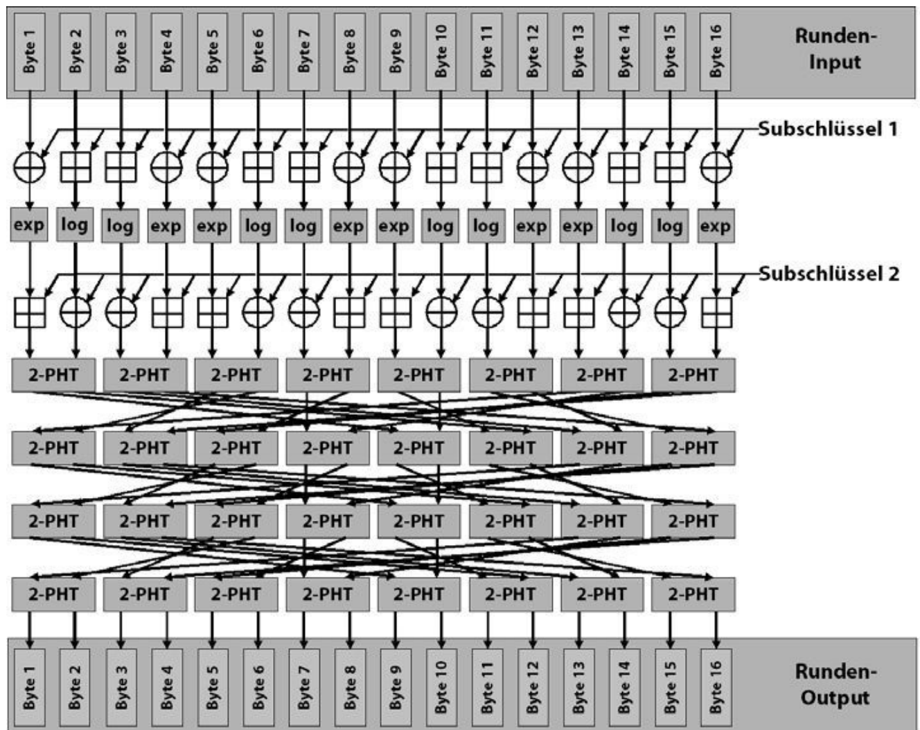
Abb. 11-5 Eine Runde des Verschlüsselungsverfahrens SAFER+. Die Rundenzahl beträgt je nach Schlüssellänge 8, 12 oder 16.
