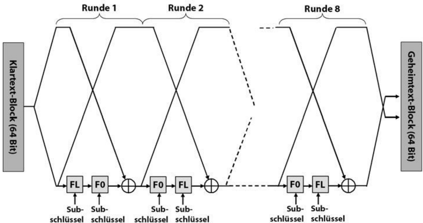
Abb. 12–1 KASUMI ist eine Feistel-Chiffre, die vor allem für Hardwareimplementierungen geeignet ist.
