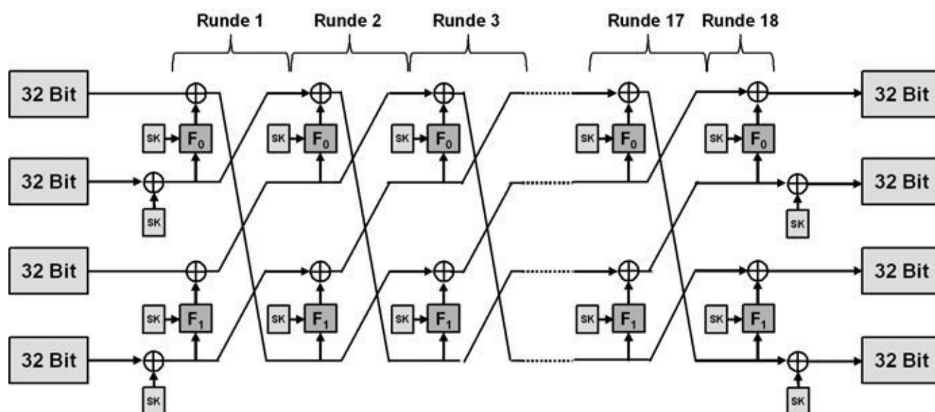
Abb. 12–3 CLEFIA ist eine verallgemeinerte Feistel-Chiffre, die für den Einsatz im Digital Rights Management entwickelt wurde.
