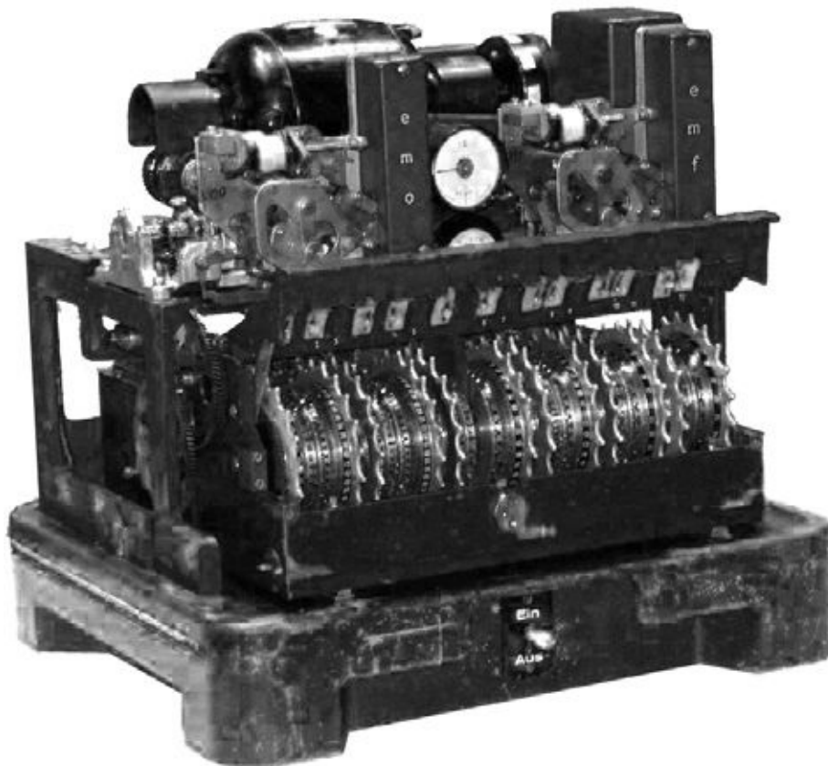
Abb. 5–15 Die Lorenz-Maschine kam auf höchster militärischer Ebene zum Einsatz. Die Briten konnten sie knacken.
