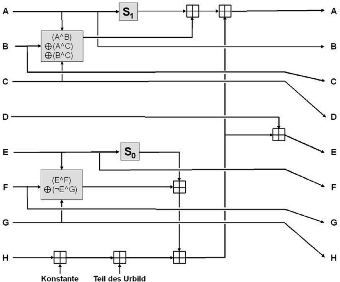
Abb. 16–4 Diese Teilrunde wird in jeder Runde von SHA-256 16-mal durchlaufen. Die Konstante ändert sich mit jeder Teilrunde.
