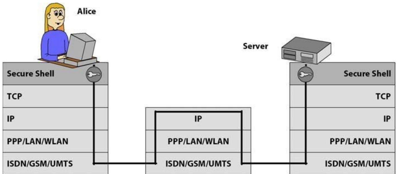
Abb. 44–3 Die Secure Shell ist eine Mehrzweck-Kryptolösung für Schicht 7.
