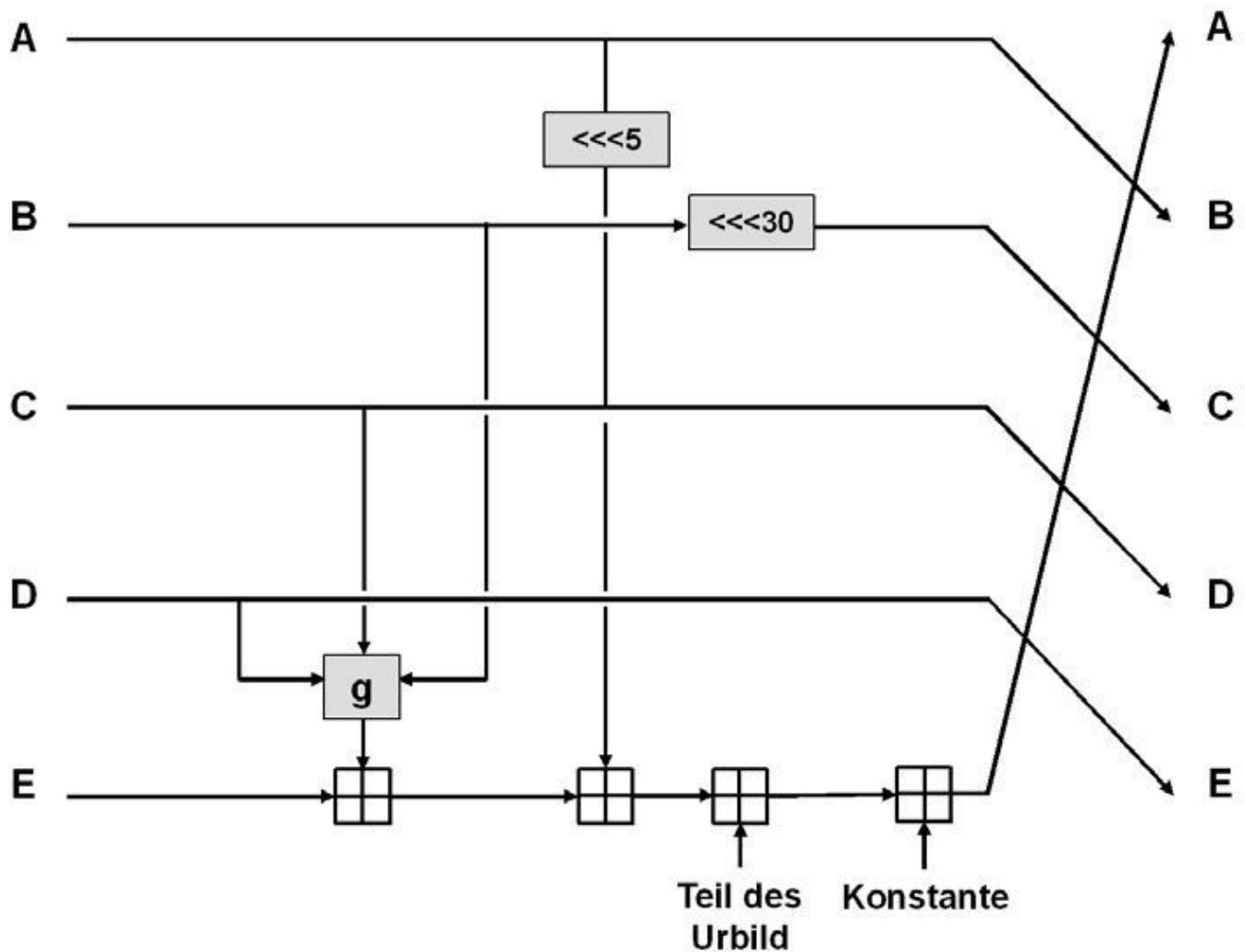
Abb. 16–3 Diese Teilrunde wird in jeder Runde von SHA-1 20-mal durchlaufen. Die Funktion g und die Konstante ändern sich mit jeder Runde.
