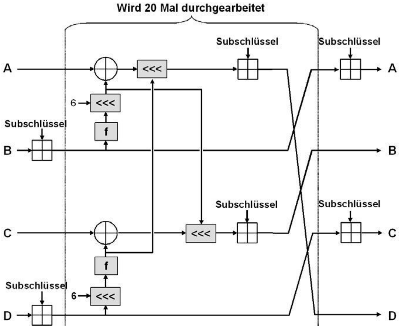
Abb. 11–4 RC6 arbeitet in 20 Runden, wobei in jede Runde zwei Subschlüssel eingehen.
