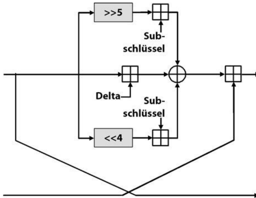
Abb. 9-4 Eine TEA-Runde. Die Zeichen »<<« und »>>« stehen für eine bitweise Verschiebung nach links bzw. rechts. Delta ist eine rundenabhängige Konstante.
