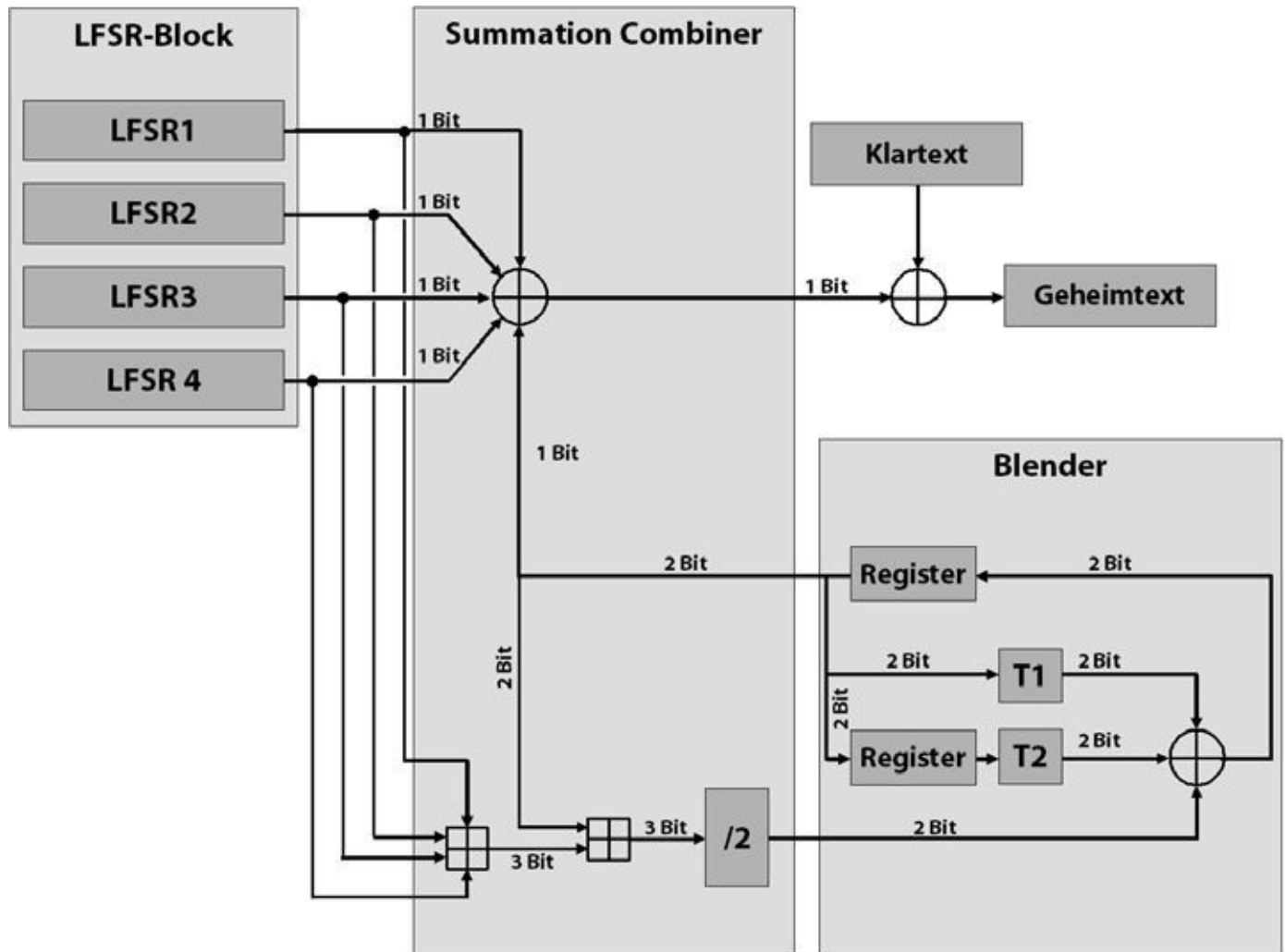
Abb. 21–3 E_0 ist eine Stromchiffre, die auf vier LFSRs basiert. Außerdem geht die Ausgabe einer zusätzlichen Komponente (Blender) in die Verschlüsselung mit ein.
