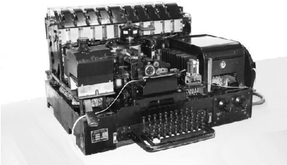
Abb. 5–12 Der Geheimschreiber (T-52) war nach der Enigma das bedeutendste deutsche Verschlüsselungsgerät des Zweiten Weltkriegs.
