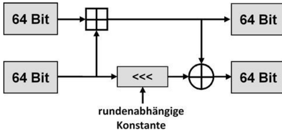
Abb. 12–7 Die Funktion MIX ist ein Bestandteil von Threefish.
