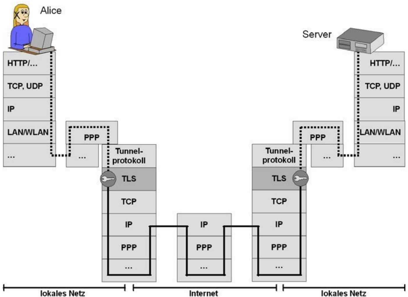
Abb. 42–3 Mit TLS lässt sich ein VPN realisieren.
