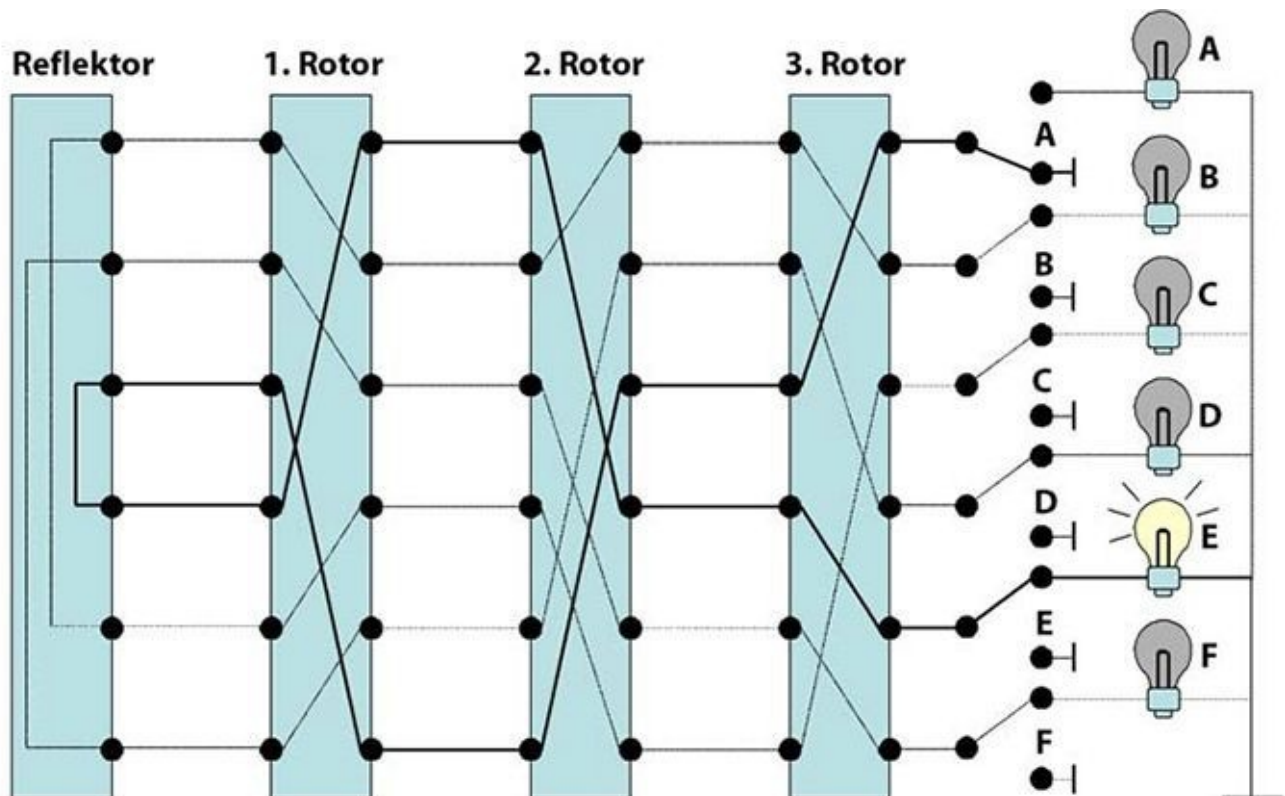
Abb. 5–4 Die Enigma realisiert eine Rotorchiffre, bei der jeder Rotor zweimal durchlaufen wird. Diese Eigenschaft wird durch den Reflektor gewährleistet, der nur auf einer Seite Kontakte hat.
