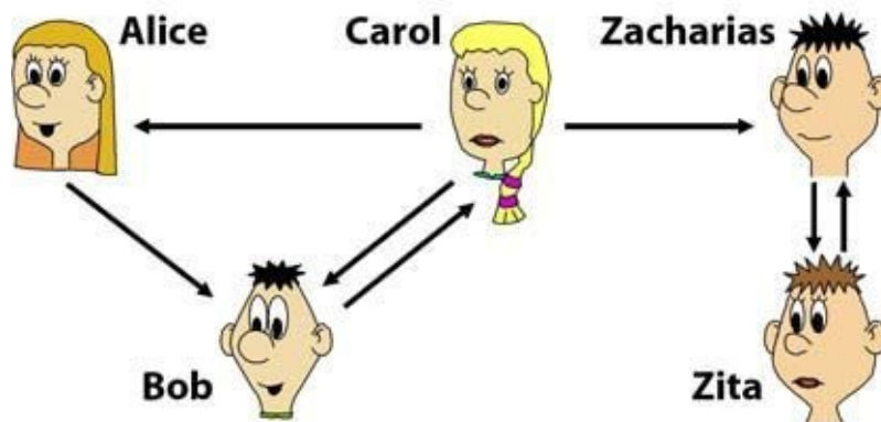
Abb. 33–2 In einem Web of Trust kann jeder für jeden Zertifikate ausstellen.
