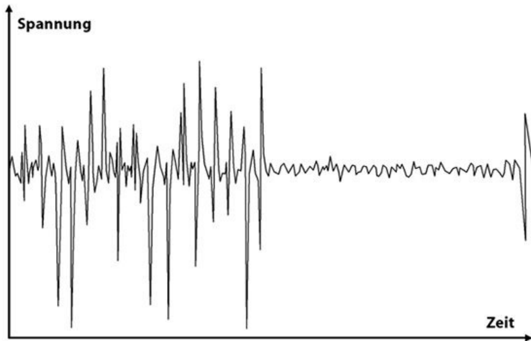
Abb. 22–2 Der Unterschied zwischen den ersten 16 Bytes (Zufallswerte) und den restlichen 16 Bytes (jeweils mit demselben Wert) ist im Oszilloskop-Bild gut zu erkennen.
