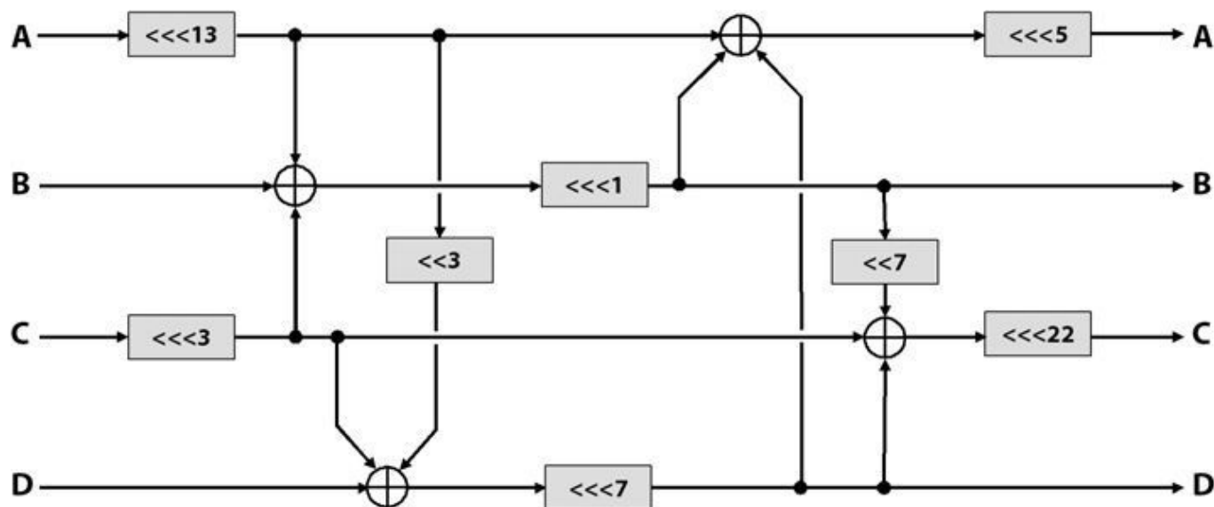
Abb. 11–2 Die lineare Transformation von Serpent arbeitet mit Linksrotationen (»<<<«) und Linksverschiebungen (»<<<«).
