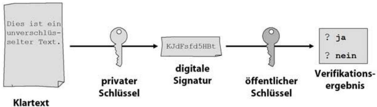
Abb. 14–1 Eine digitale Signatur wird mit einem privaten Schlüssel erzeugt. Die Überprüfung der Echtheit erfolgt mit dem zugehörigen öffentlichen Schlüssel.
