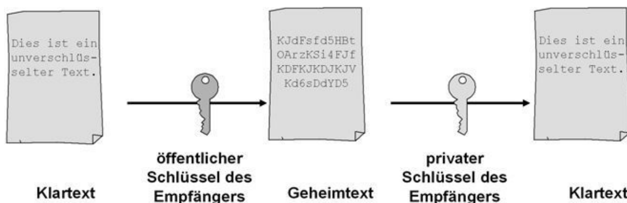
Abb. 13–2 So funktioniert eine Public-Key-Verschlüsselung: Zum Verschlüsseln wird ein anderer Schlüssel verwendet als zum Entschlüsseln. Ersterer ist öffentlich bekannt. Letzterer wird vom Empfänger geheim gehalten, weshalb man ihn privaten Schlüssel nennt.
