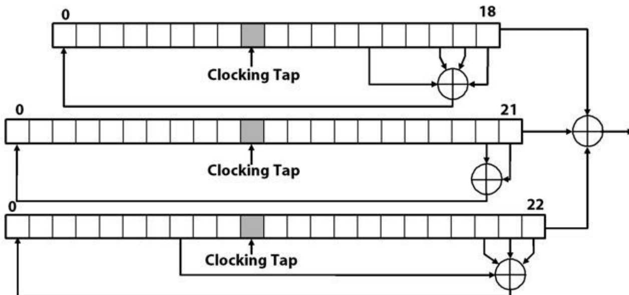
Abb. 21–2 Funktionsweise des Verschlüsselungsverfahrens A5. Es sieht drei LFSRs vor, deren Ausgabe mit dem Klartext verknüpft wird. Inzwischen ist bekannt, dass es sich dabei um ein vergleichsweise schwaches Verfahren handelt.
