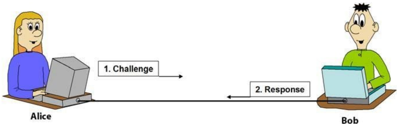
Abb. 26–6 Bei einem Challenge-Response-Verfahren hat Mallory keine Möglichkeit, das Passwort abzuhören.
