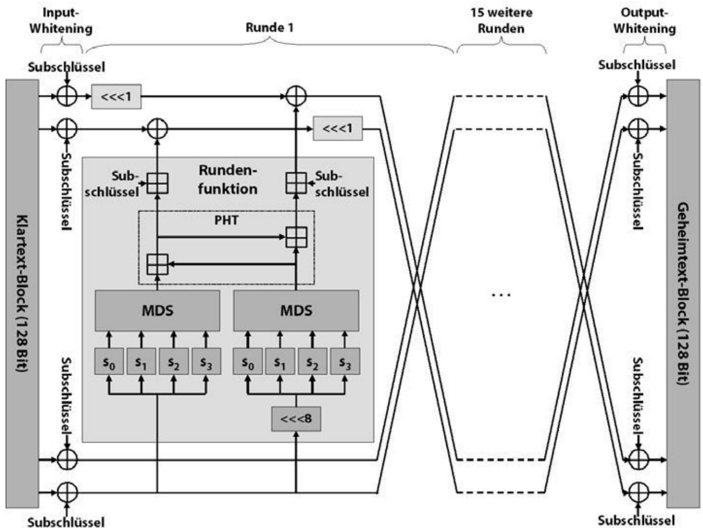
Abb. 11-3 Twofish ist eine Feistel-Chiffre mit 16 Runden. Die Schlüssellänge beträgt 128, 192 oder 256 Bit.
