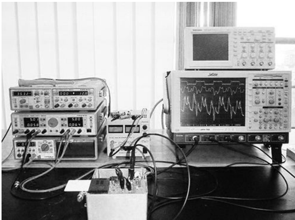
Abb. 22–1 Für einen Stromangriff benötigt Angreifer Mallory eine geeignete Ausrüstung. Dazu gehört insbesondere ein Speicheroszilloskop. (Quelle: cryptovision)
