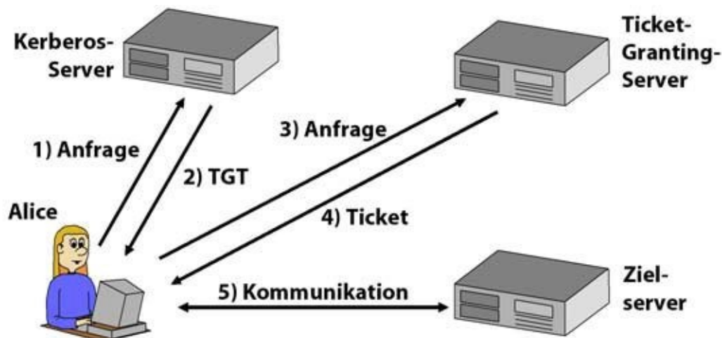
Abb. 27-2 Kerberos ermöglicht ein ticketbasiertes Single Sign-on ohne asymmetrische Kryptografie.
