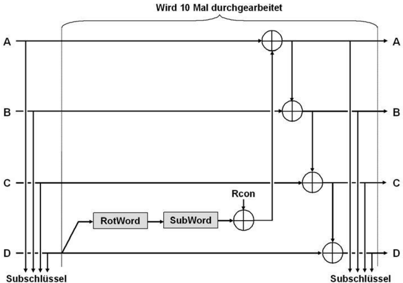
Abb. 10–1 Die AES-Schlüsselaufbereitung generiert für die 128-Bit-Variante 11 Subschlüssel.
