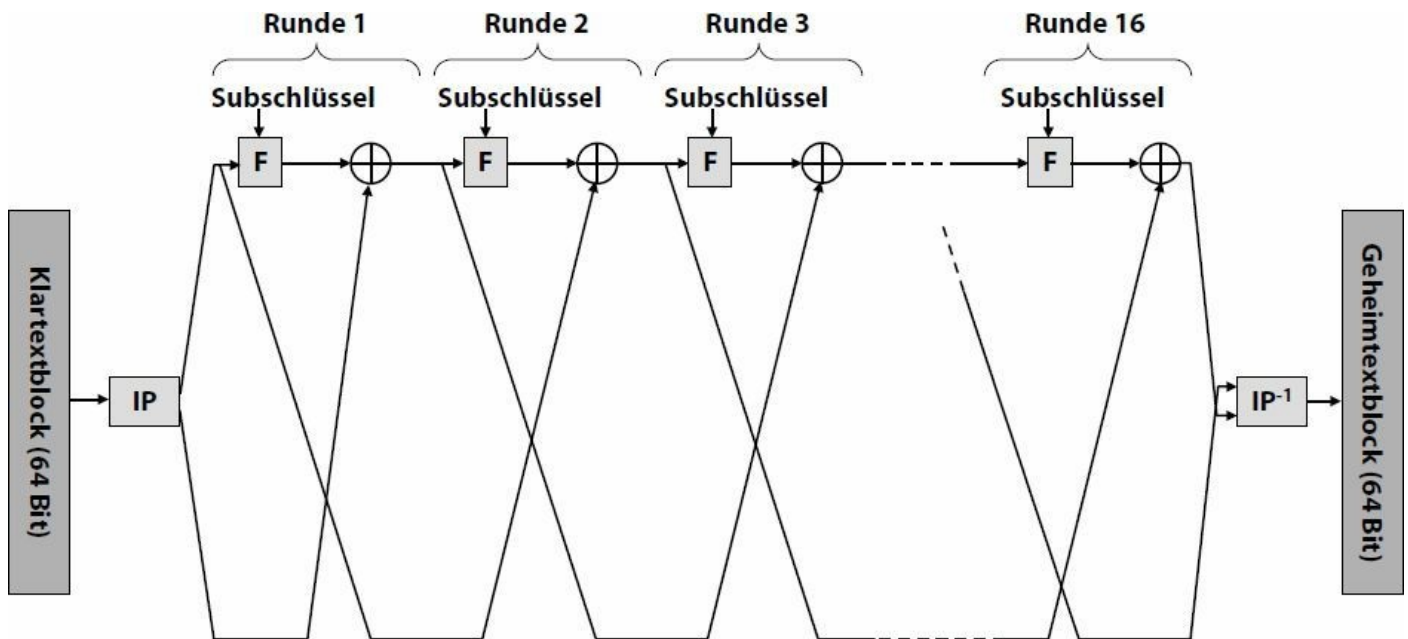
Abb. 6–1 Der DES sieht 16 Runden vor, in die jeweils ein Subschlüssel eingeht. Der Aufbau der Funktion F wird im nächsten Bild erklärt.
