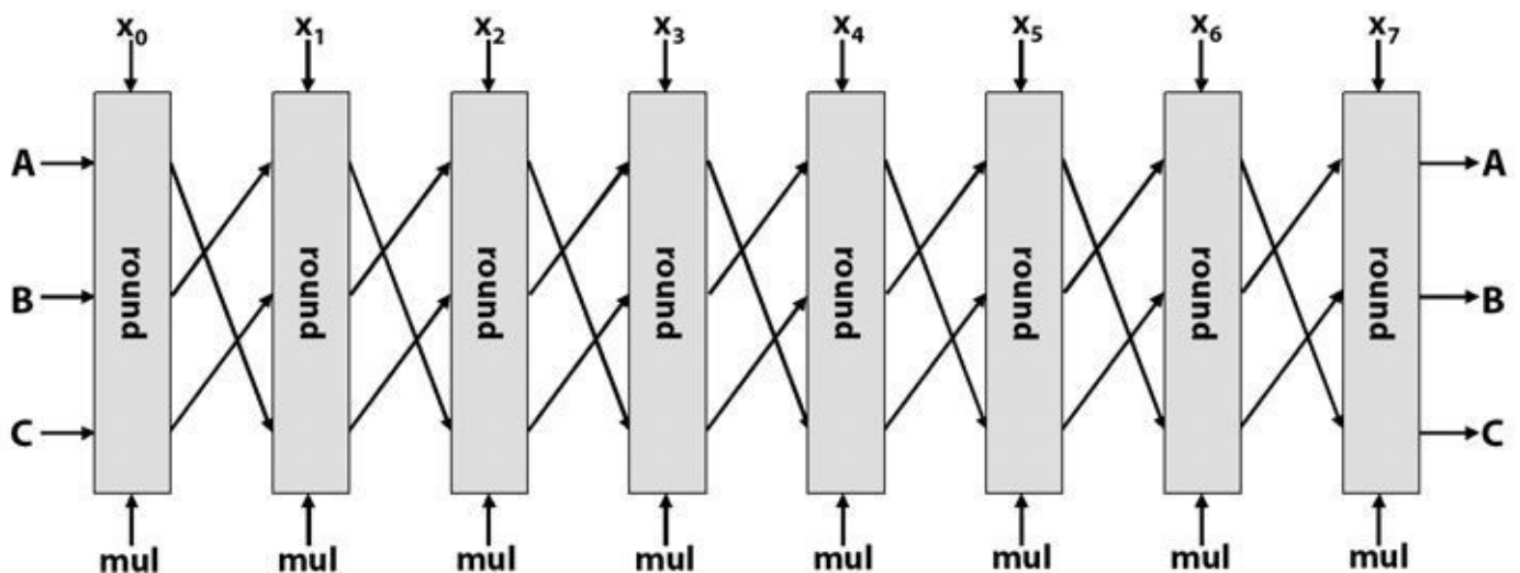
Abb. 17-3 Jede Tiger-Runde besteht aus acht Teilrunden, die round genannt werden. x_0, x_1, \dots, x_7 ist ein Urbild-Block. Die Variable mul kann die Werte 5, 7 und 9 annehmen.
