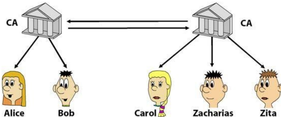
Abb. 33–6 Bei einer Cross-Zertifizierung stellen sich zwei CAs gegenseitig je ein Zertifikat aus.
