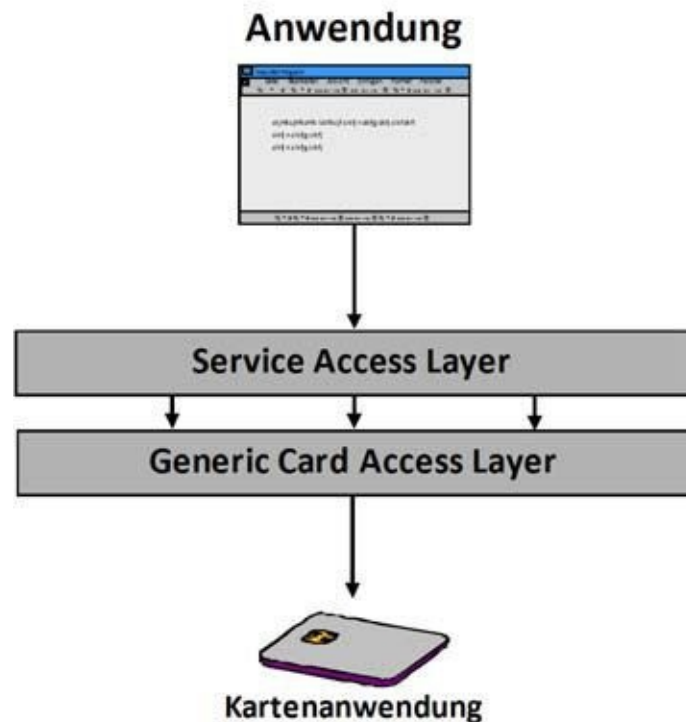
Abb. 31–3 ISO/IEC 24727 ist eine Krypto-API, die vor allem für elektronische Ausweise geeignet ist.
