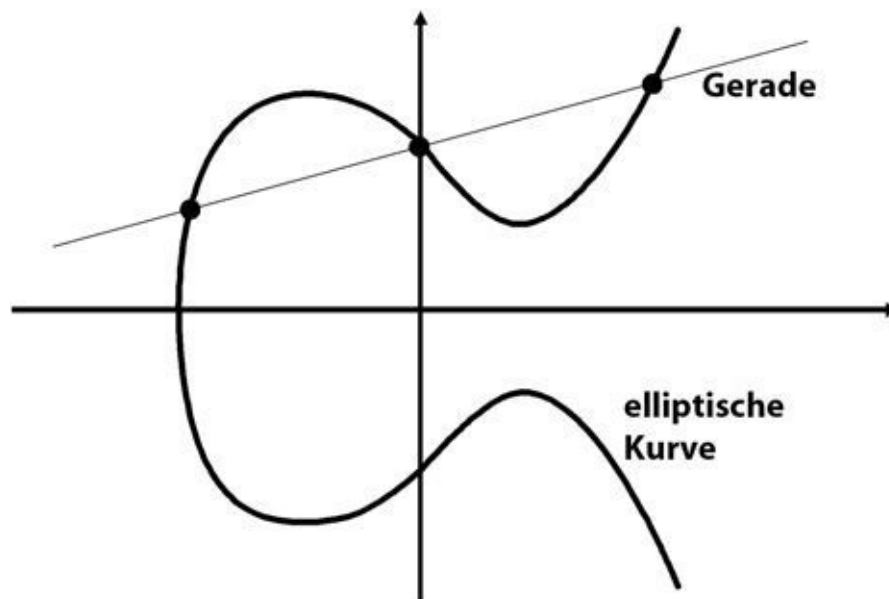
Abb. 15–1 Lässt man einige Spezialfälle außen vor, dann gilt: Eine Gerade schneidet eine elliptische Kurve in genau drei Punkten.
