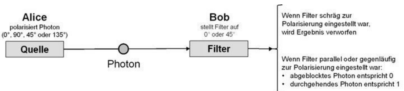
Abb. 29–1 Mithilfe von Photonen können Alice und Bob auf beweisbar sichere Weise einen Schlüssel vereinbaren. Angreifer Mallory müsste zum Mitlesen selbst einen Filter aufstellen, mit dem er jedoch die Polarisierung der Photonen ändern würde – und das würde auffallen.
