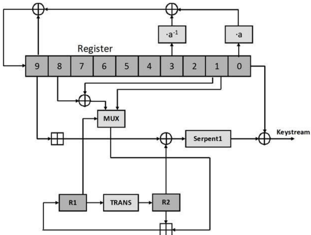
Abb. 21–10 Die Stromchiffre Sosemanuk arbeitet mit einem Status, der aus insgesamt zwölf 32-Bit-Variablen besteht. Zehn davon bilden das Register, die zwei verbleibenden heißen R1 und R2 .
