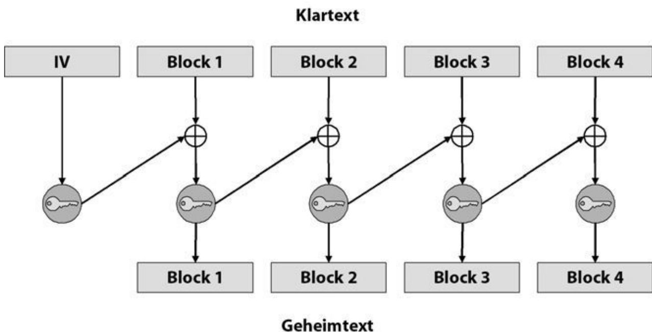
Abb. 24-3 Im CBC-Modus wird jeder Klartextblock mit dem letzten Geheimtextblock verknüpft.
