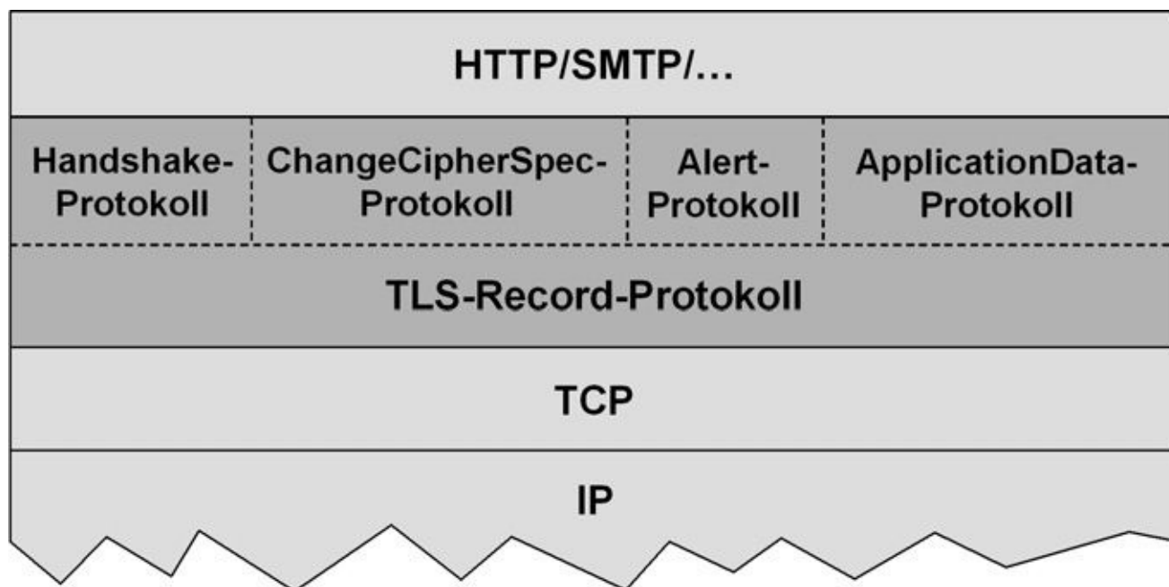
Abb. 42–2 TLS gliedert sich in zwei Teilschichten. Die obere ist für das Aushandeln von Verfahren und Fehlermeldungen zuständig. Die untere Schicht übernimmt die Verschlüsselung.
