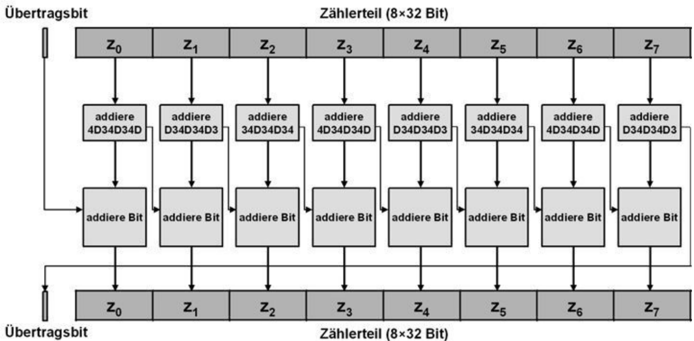
Abb. 21–7 Der Zählerteil von Rabbit wird mit linearen Funktionen fortgeschaltet.
