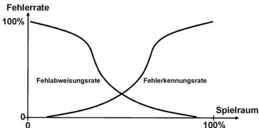
Abb. 26–2 Verlauf der Fehlerkennungs- und der Fehlabweisungsrate bei einem Biometriesystem
