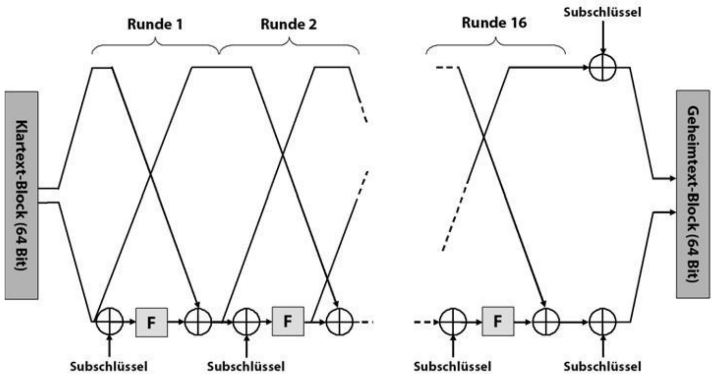
Abb. 9–3 Blowfish arbeitet in 16 Runden. Das Design des Verfahrens ähnelt in einigen Punkten dem DES, wobei jedoch schlüsselabhängige S-Boxen zum Einsatz kommen.
