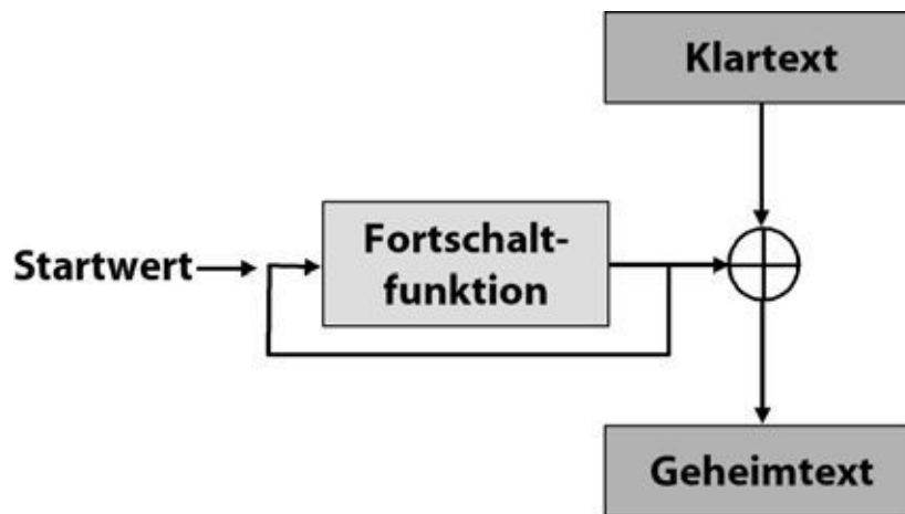
Abb. 21–1 Bei einer Stromchiffre wird die Ausgabe eines Pseudozufallsgenerators mit dem Klartext verknüpft.
