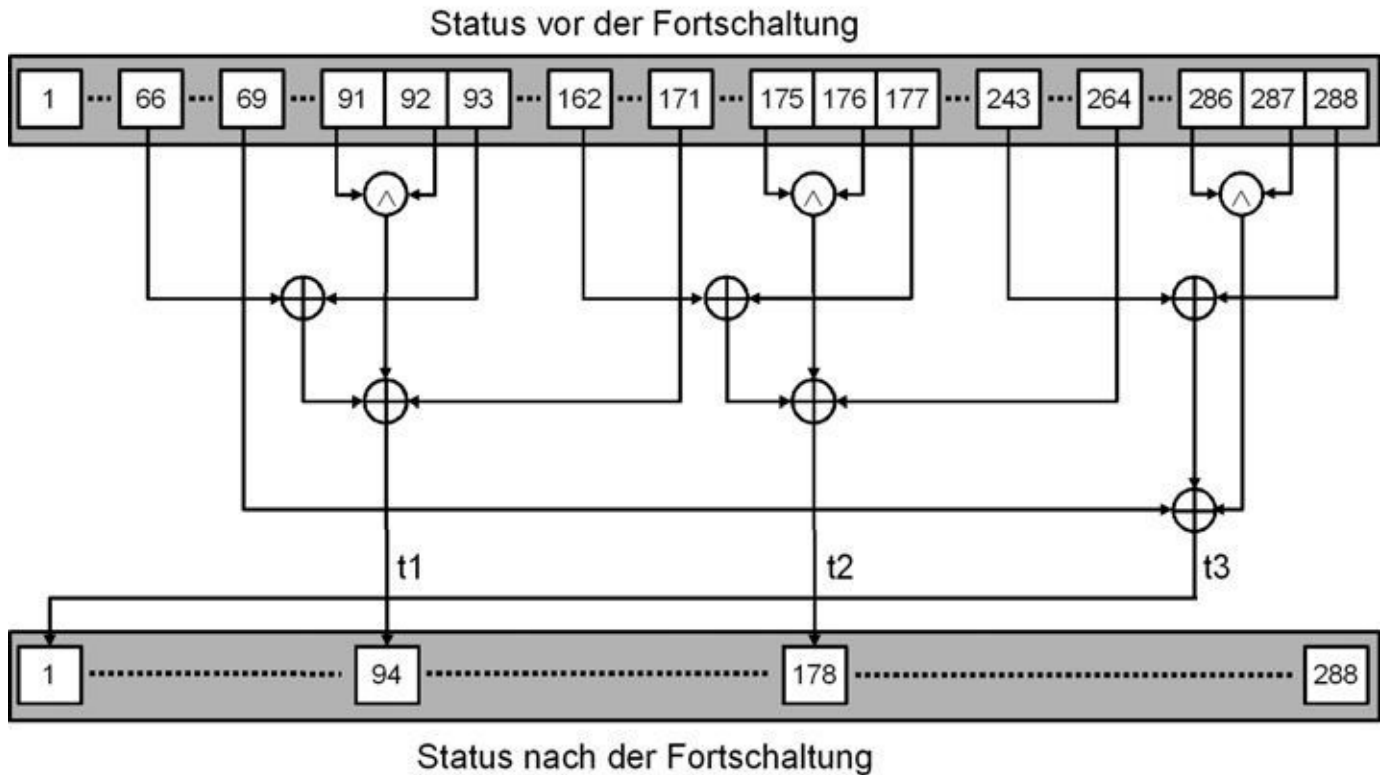
Abb. 21–12 Trivium erhielt im Rahmen des eSTREAM-Wettbewerbs hervorragende Beurteilungen. Das für Hardwareumgebungen gedachte Verfahren ist einfach und gilt als sicher.
