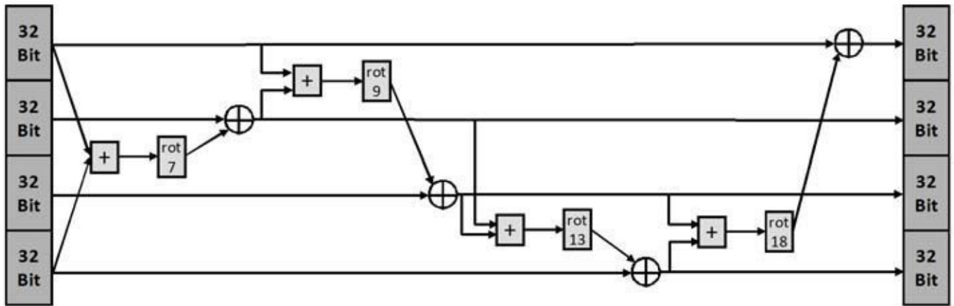
Abb. 21–9 Die Viertelrundenfunktion ist der zentrale Bestandteil von Salsa20. Sie spielt bei der Keystream-Generierung eine Rolle.
