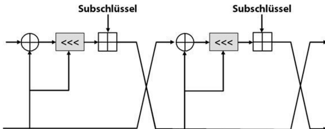
Abb. 9–2 Eine Runde von RC5 entspricht zwei Feistel-Runden. Die Sicherheit des Verfahrens hängt zu einem wesentlichen Teil von datenabhängigen Rotationen ab.
