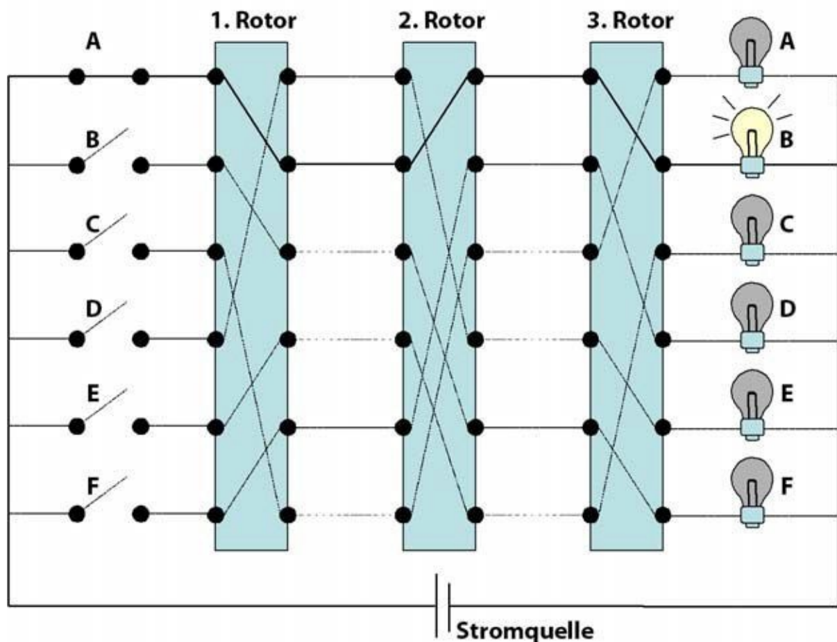
Abb. 5–2 Eine Rotorchiffre mit drei Rotoren (statt 26 sind nur sechs Buchstaben abgebildet): Wird die »A«-Taste gedrückt, dann leuchtet durch die Verdrahtung die »B«-Lampe auf. Da sich die Rotoren drehen, ändert sich der Weg des Stroms ständig.
