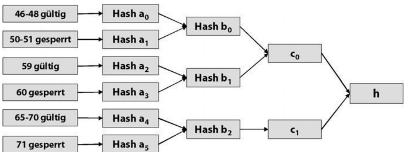
Abb. 35–1 Beispiel für einen Sperrbaum. Je mehr Zertifikate gesperrt sind, desto mehr lohnt es sich, statt mit Sperrlisten mit Sperrbäumen zu arbeiten.
