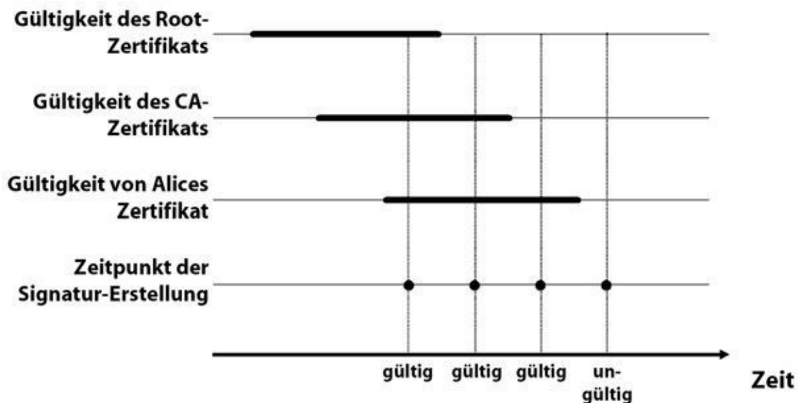
Abb. 36–3 Das Kettenmodell ist das wichtigste Gültigkeitsmodell.
