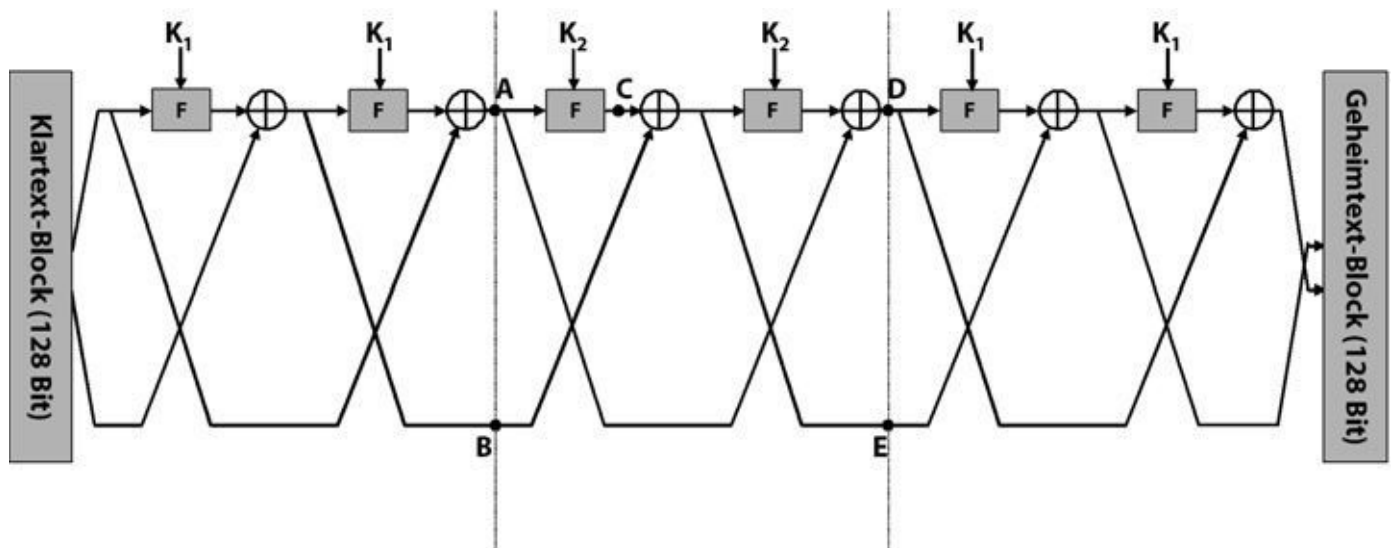
Abb. 11–6 MAGENTA ist eine Feistel-Chiffre mit einer Schwäche in der Schlüsselaufbereitung.
