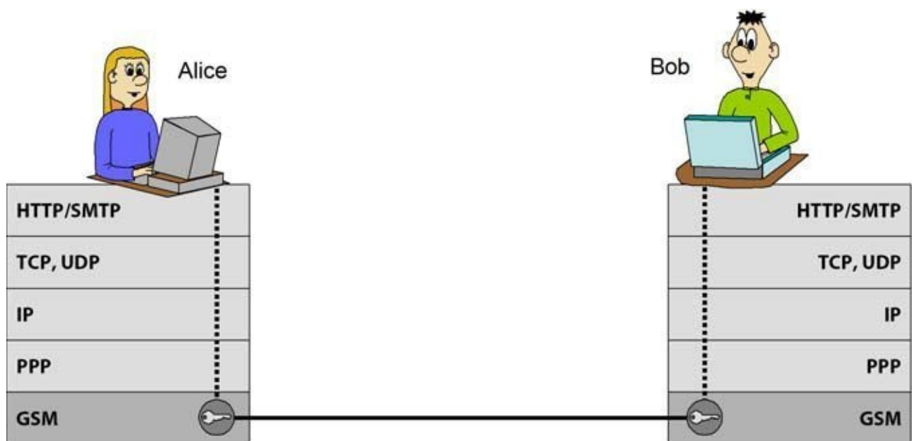
Abb. 39-2 Auch GSM dient im Internet als Schicht-1-Protokoll. GSM war eines der ersten Protokolle, bei dem kryptografische Mechanismen fest eingebaut waren.
