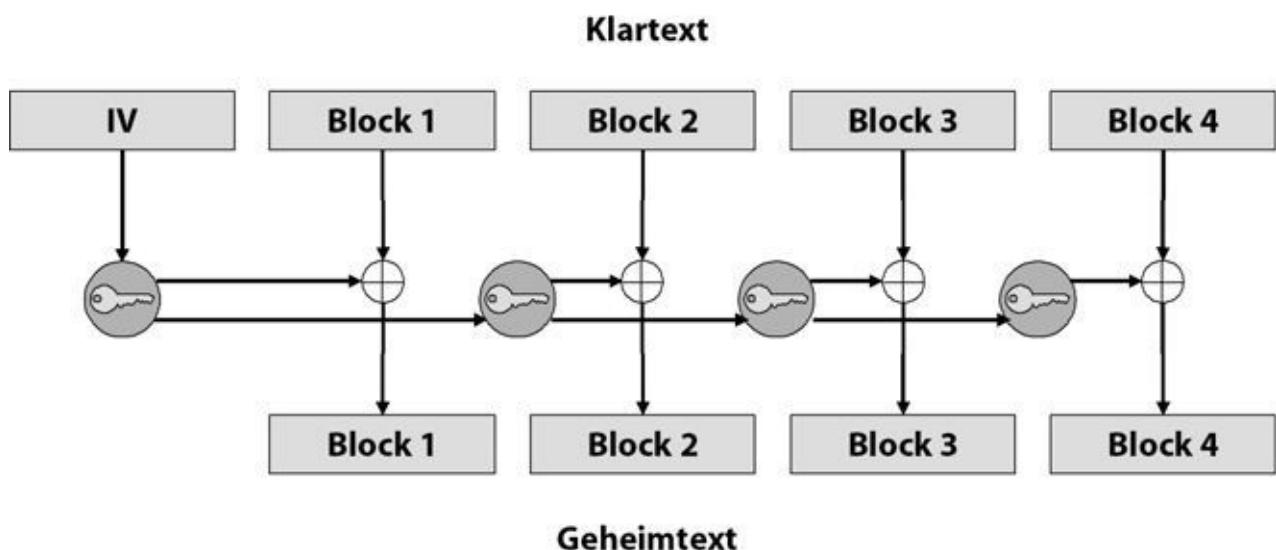
Abb. 24–4 Im OFB-Modus wird eine Blockchiffre als Stromchiffre betrieben.
