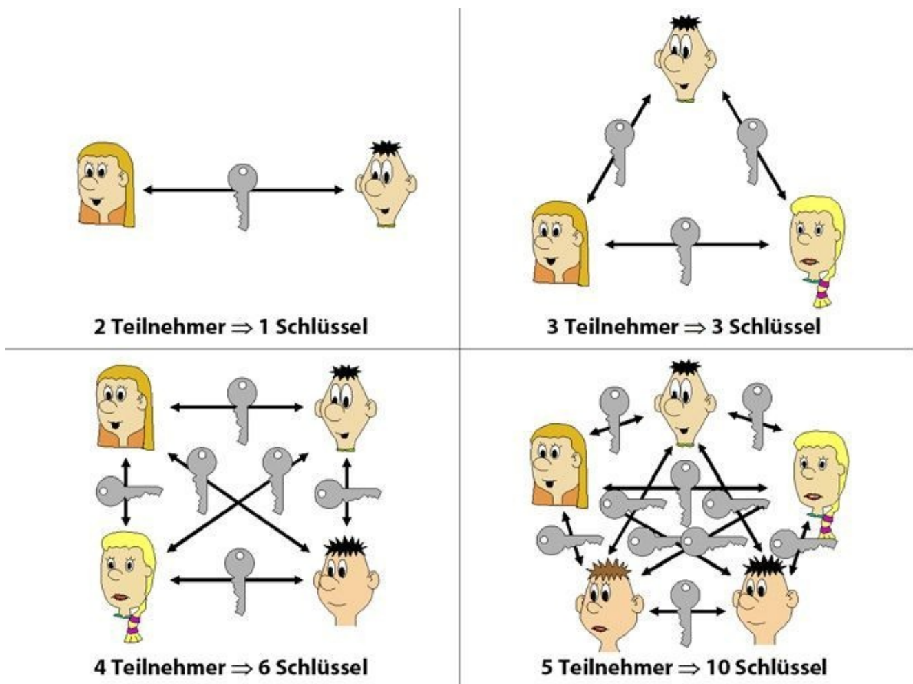
Abb. 13–1 Um ein symmetrisches Verschlüsselungsverfahren einzusetzen, müssen je zwei Teilnehmer einen gemeinsamen geheimen Schlüssel besitzen. Dies ist nur bei kleineren Teilnehmerzahlen sinnvoll, da sonst die Anzahl der Schlüssel zu groß wird.
