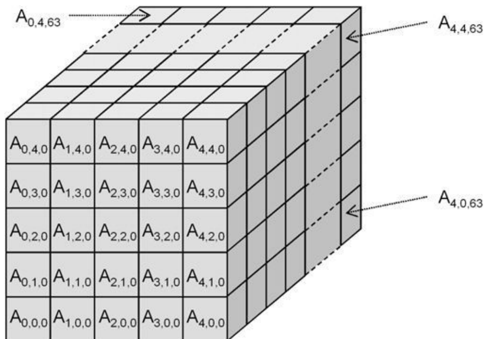
Abb. 17–6 Der Status von Keccak ist ein dreidimensionales Array bestehend aus 5x5x64 Bits.
