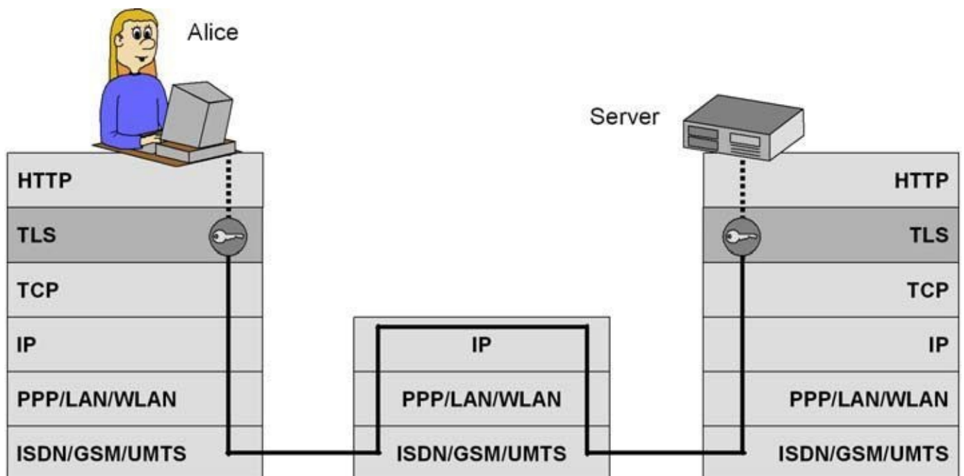
Abb. 44–2 Wird HTTP zusammen mit TLS eingesetzt, so nennt man dieses Protokollpaar HTTPS.
