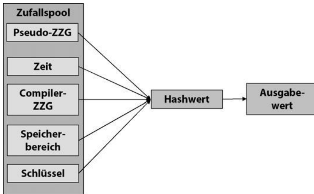
Abb. 19–2 Das Mischen von Zufallszahlen unterschiedlicher Herkunft mit einer Hashfunktion gilt als gute Methode zur Generierung von Zufallsfolgen.
