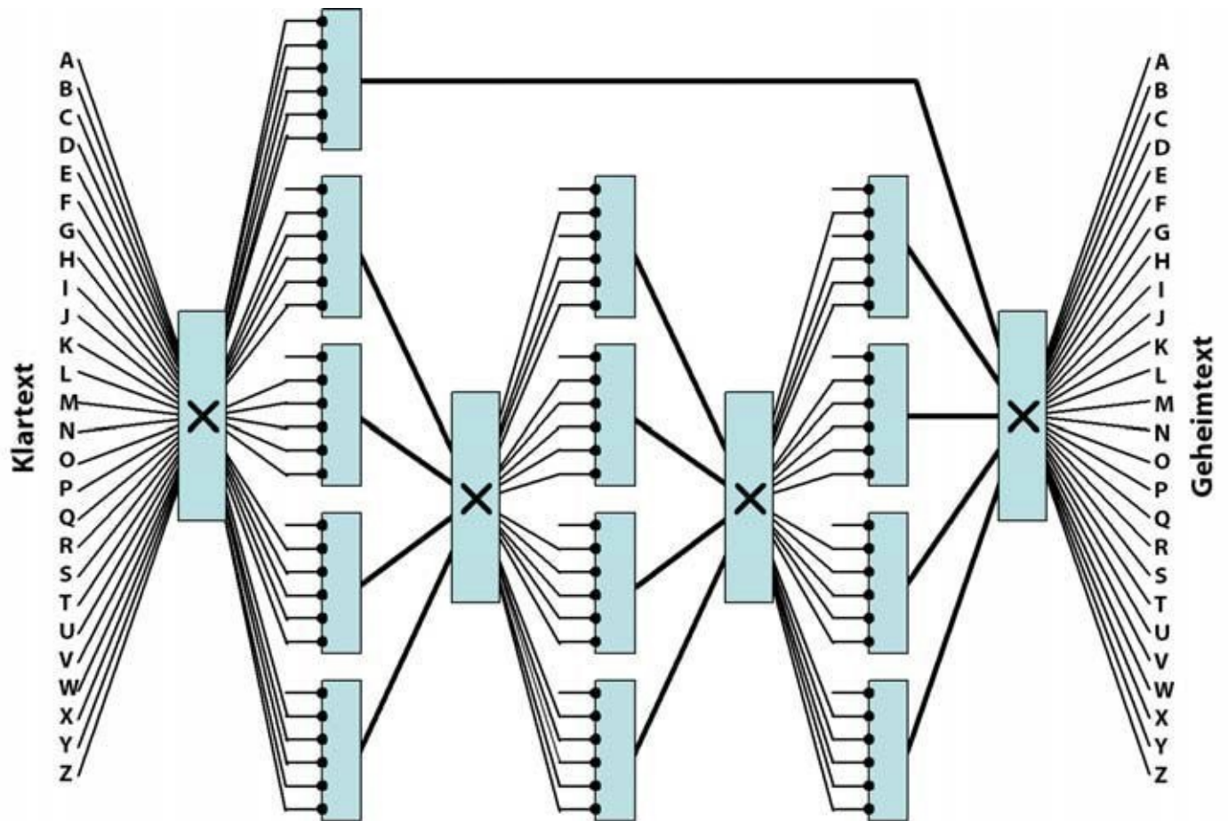
Abb. 5–11 Die Purple arbeitete mit 13 Telefon-Vermittlungsschaltern, die je sechs Eingänge hatten (teilweise blieb einer davon ungenutzt). In jedem Schalter verbanden sechs Zeiger die Eingänge mit 150 Ausgängen. Zeiger und Ausgänge sind hier nicht abgebildet.
