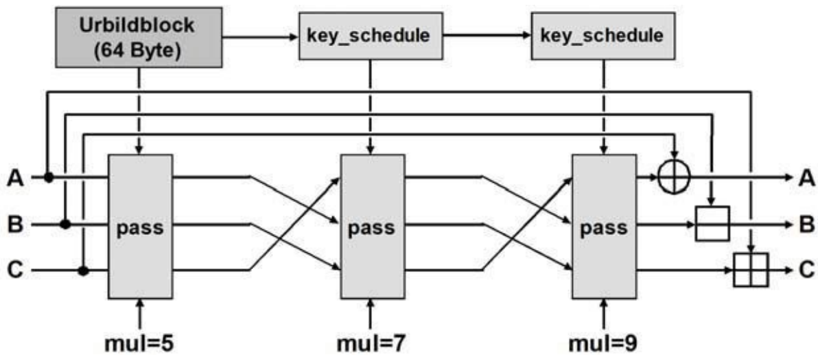
Abb. 17–1 Die Kompressionsfunktion von Tiger sieht drei Runden vor, die als pass bezeichnet werden.
