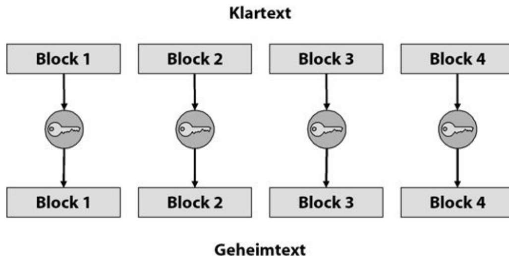
Abb. 24–1 Im ECB-Modus wird jeder Klartextblock unabhängig von den anderen verschlüsselt. ECB ist damit die einfachste Betriebsart.
