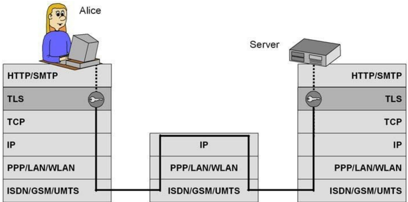
Abb. 42–1 TLS setzt zwischen TCP und einem Anwendungsprotokoll wie HTTP oder SMTP an. Das Anwendungsprotokoll und die Anwendungssoftware müssen nicht geändert werden.
