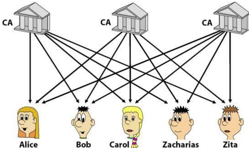
Abb. 33–5 Im Webmodell gibt es mehrere CAs, die Zertifikate ausstellen. Ein Benutzer kann dabei mehrere Zertifikate von unterschiedlichen CAs besitzen.
