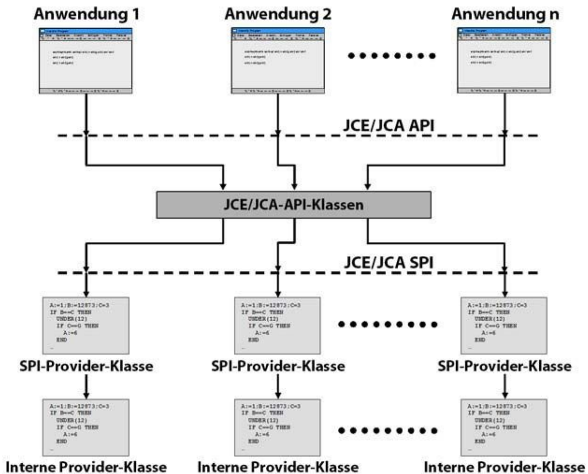
Abb. 31–5 JCA/JCE ist eine Architektur, die eine Krypto-API auf Basis von Java vorsieht.
