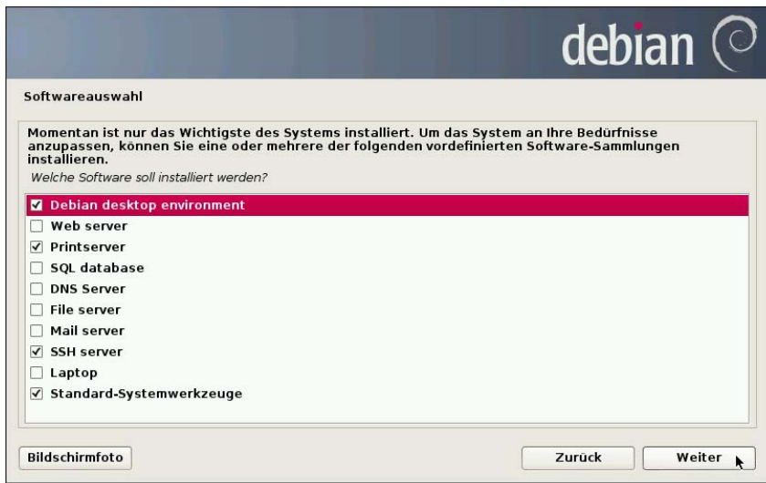
Abbildung 3.14 Wählen Sie eine oder mehrere Paketgruppen aus.
