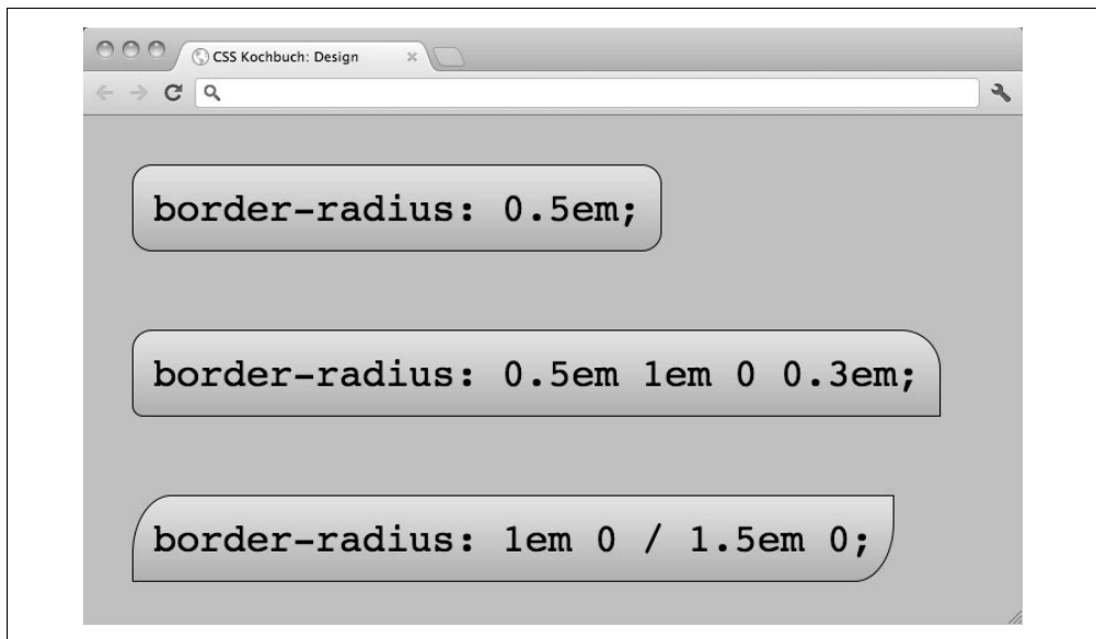
Abbildung 12-7: Elemente mit abgerundeten Ecken
