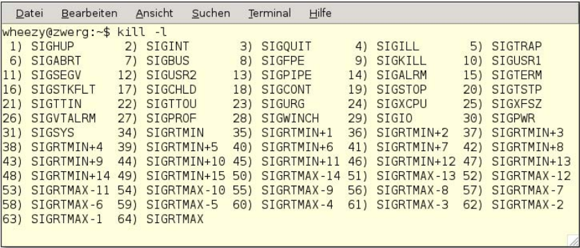
Abbildung 17.10 Das Kommando »kill -l« zeigt die möglichen Signale an.
