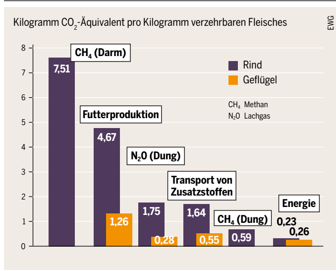
Emissionen bei der Produktion von Fleisch in den USA
