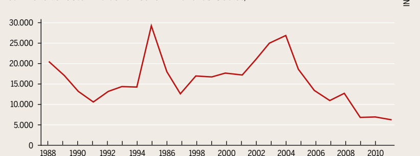
Jährliche Verluste im brasilianischen Amazonas-Gebiet, in km²
