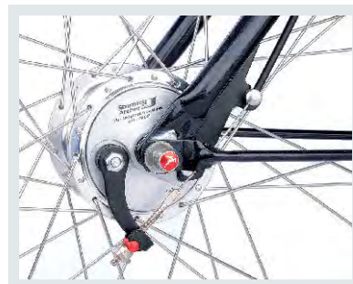
Trommelbremse
