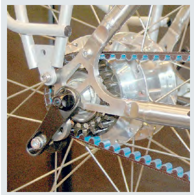
Der Snubber verhindert bei der Rohloff-Schaltung das Abspringen des Riemens.
