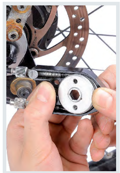
Die Seiltrommelinnenseite muss bei Rohloff Speedhub 500/14 bei Bedarf überprüft und gereinigt werden.
