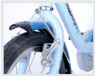
Cantilever-Bremse (neue Bauform)
